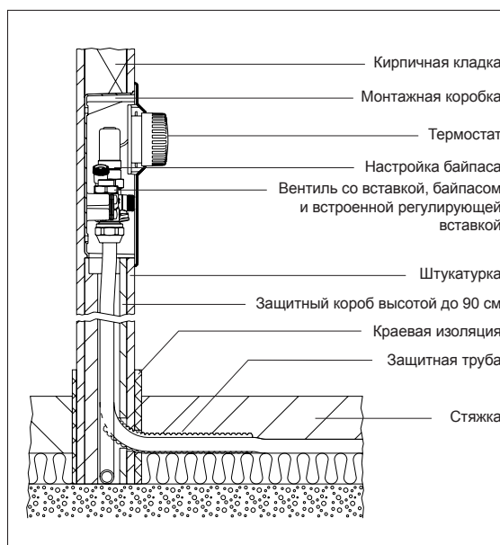
Пример установки „Unibox E BV“ в стене
