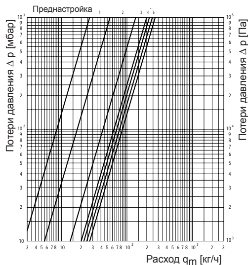
Диаграмма потерь давления „Unibox RTL“
