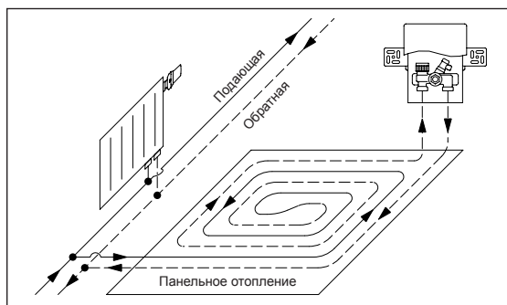
Схема монтажа „Unibox vario“, базовая модель
