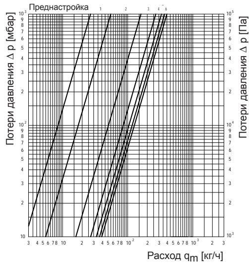
Диаграмма потерь давления как и выше, вставка AV6 при P-отклонении 1 К
