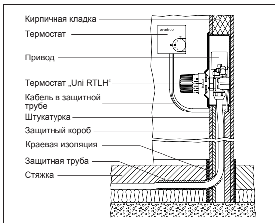
„Unibox vario“ с термостатом и приводом
