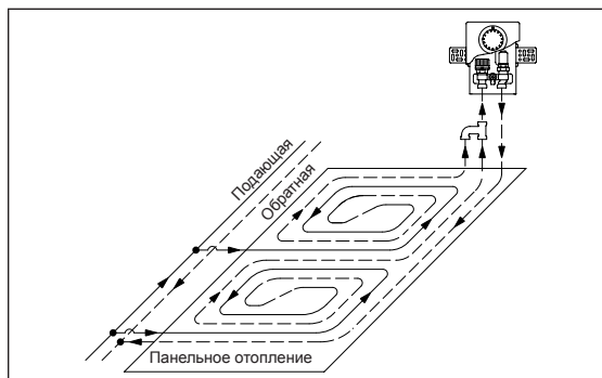
Схема „Unibox“, с двумя равными отопительными контурами
