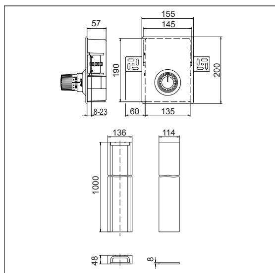
Размеры „Unibox“, глубиной 57 мм и защитного короба
