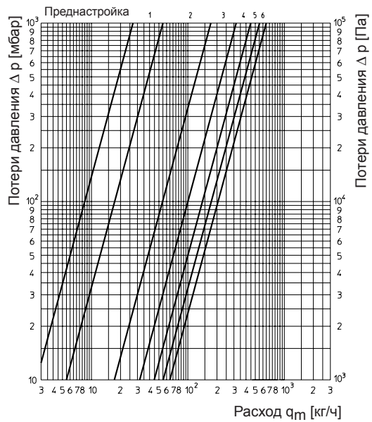
Диаграмма потерь давления для „Unibox T“, при Р-отклон. 1К и „Unibox plus“, вентиль RTLH полностью открыт
