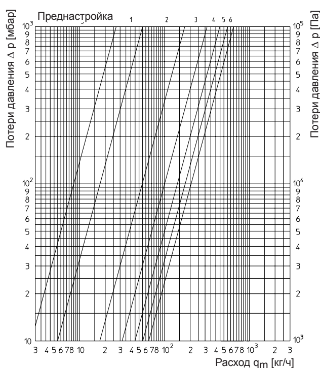
Показатели пропускной способности „Unibox T” и „Unibox plus”
