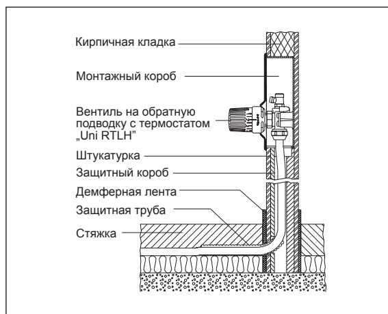
„Unibox RTL”, строительная глубина 57 мм
