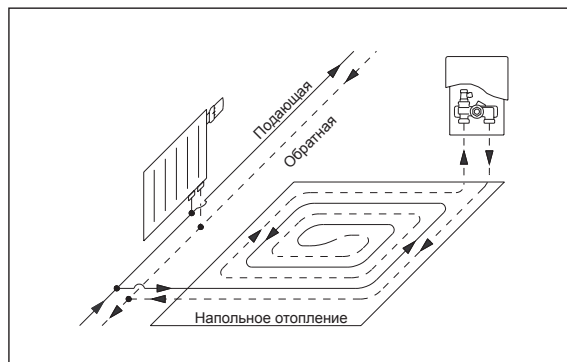
Схема монтажа: ограничение т-ры обратного потока
