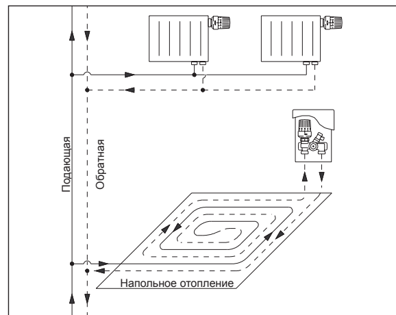
Схема регулирования температуры отдельного помещения и ограничение температуры обратного потока при напольном отоплении
