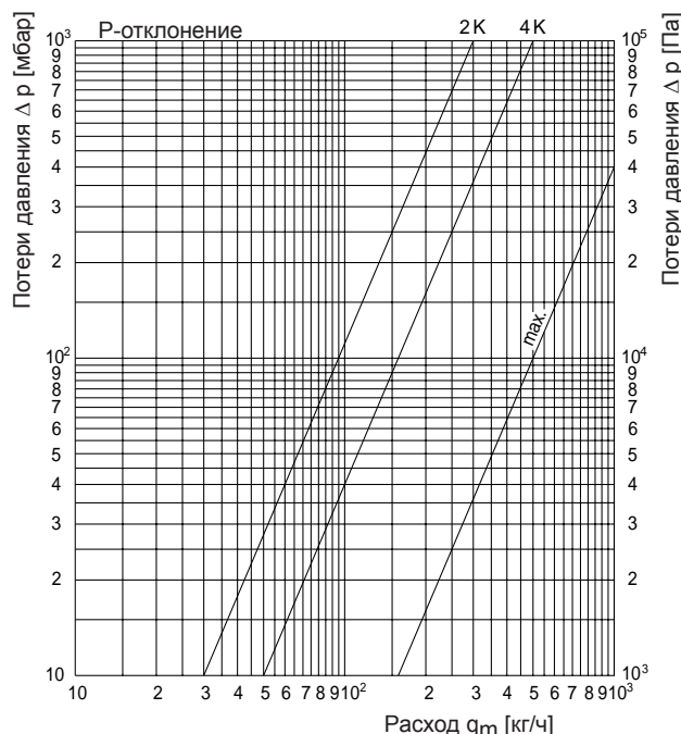
Диаграмма потерь давления „Unibox RTL”
