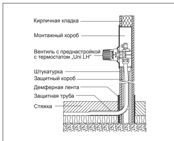
„Unibox T”, строительная глубина 57 мм
