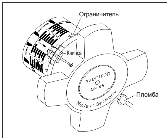
Рис. 3: блокировка и пломбировка настройки
