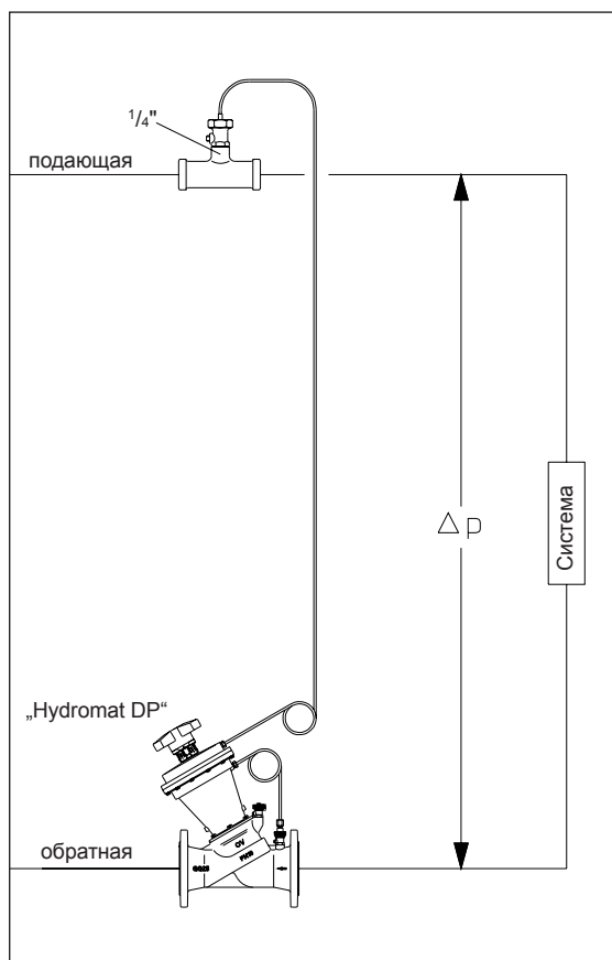
Рис. 1: „Hydromat DP”
