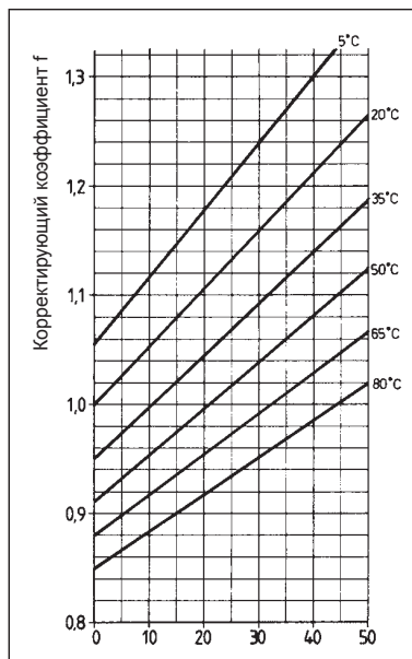
Процент этиленгликоля в смеси [%]
