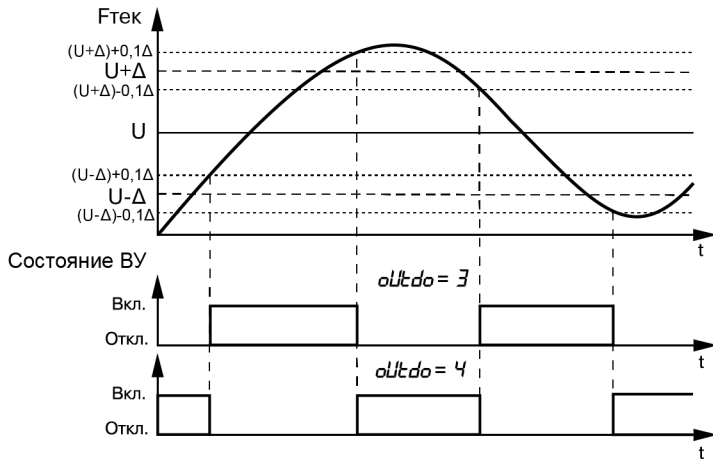
Рисунок 7.7 – Типы логики (П- и I-образная) при работе ВУ в качестве компаратора
