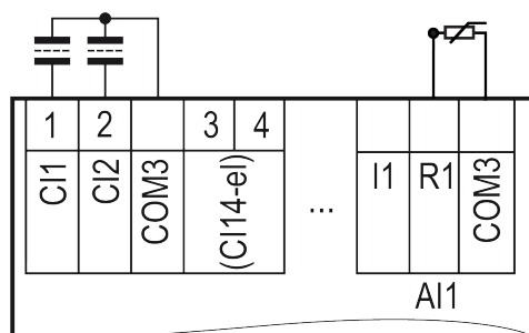
Рисунок 8.7 – Двухэлектродная схема подключения кондуктометрического датчика с коррекцией температуры
