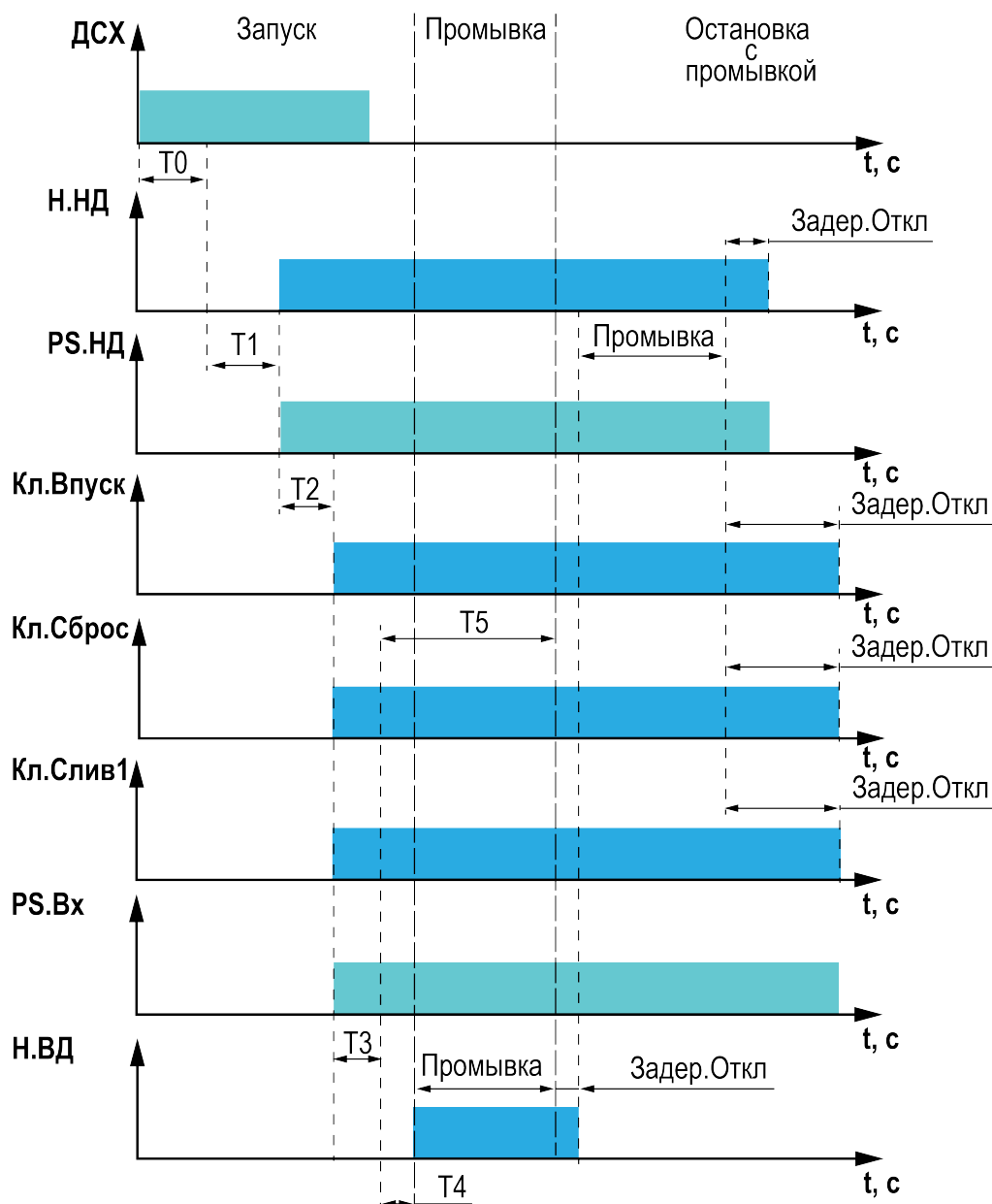
Рисунок 8.5 – Промывка в ожидании высоким давлением с промывкой при остановке низким давлением
