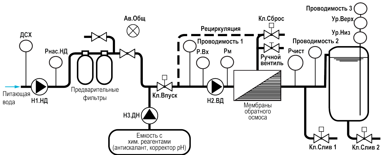
Рисунок 1.3 – Объект управления КосМастер-Х.03
