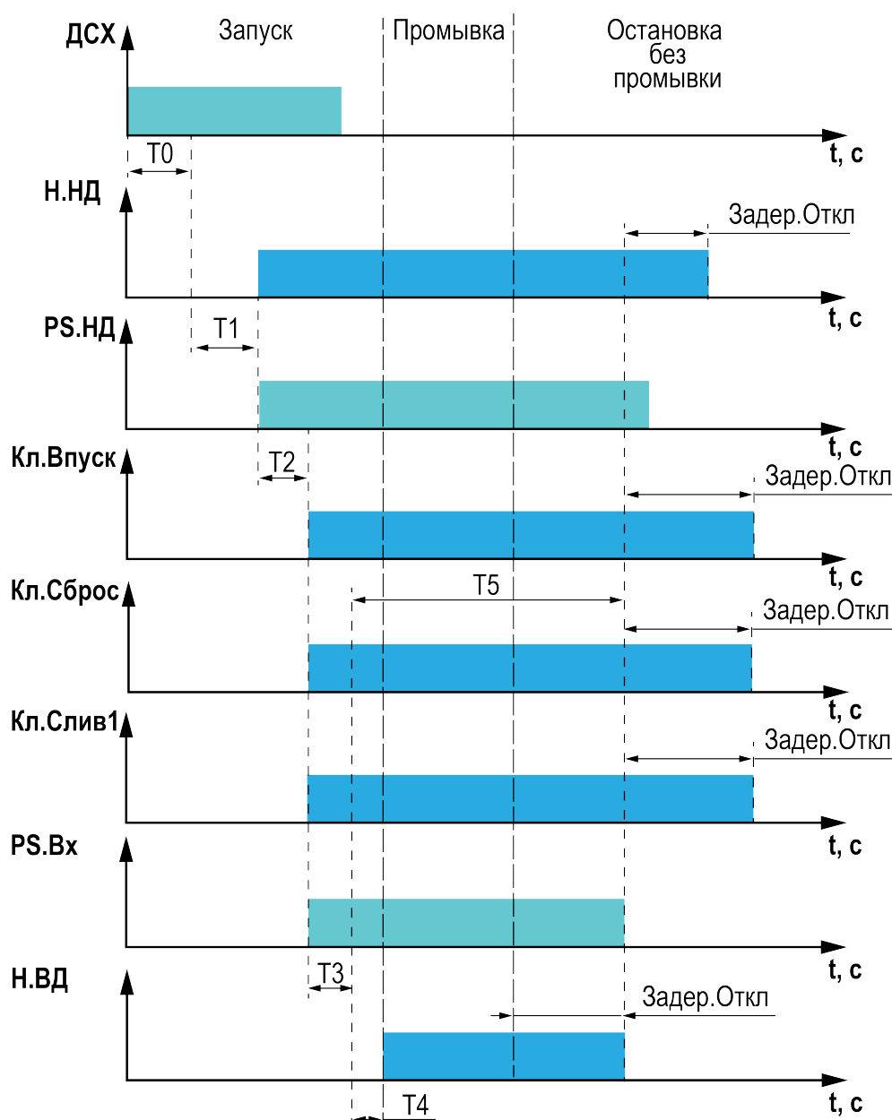
Рисунок 8.6 – Промывка в ожидании высоким давлением с отключенной промывкой при остановке
