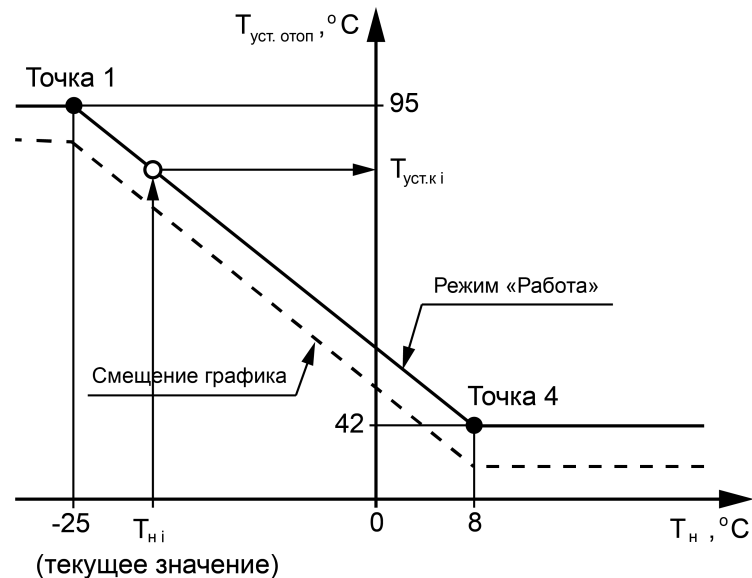
Рисунок 9.6 – Отопительный график
