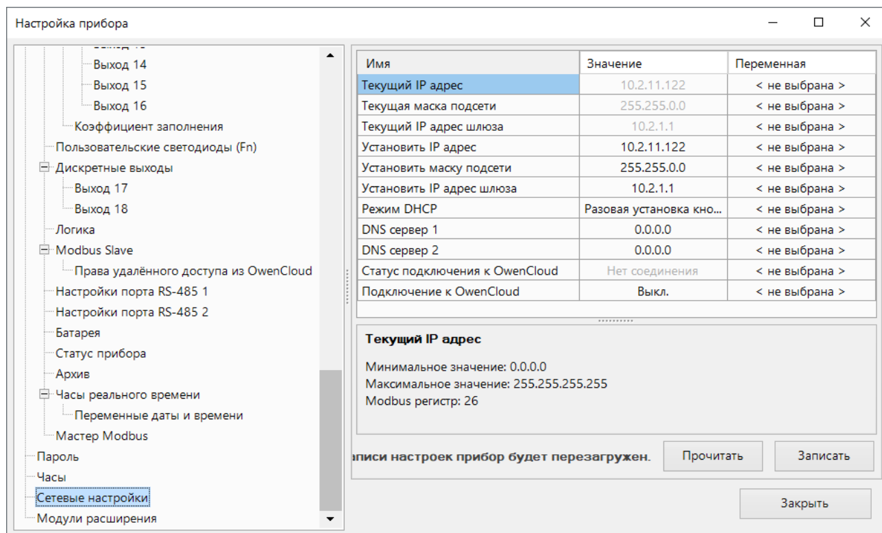
Рисунок 4.22 – Настройки параметров Ethernet
