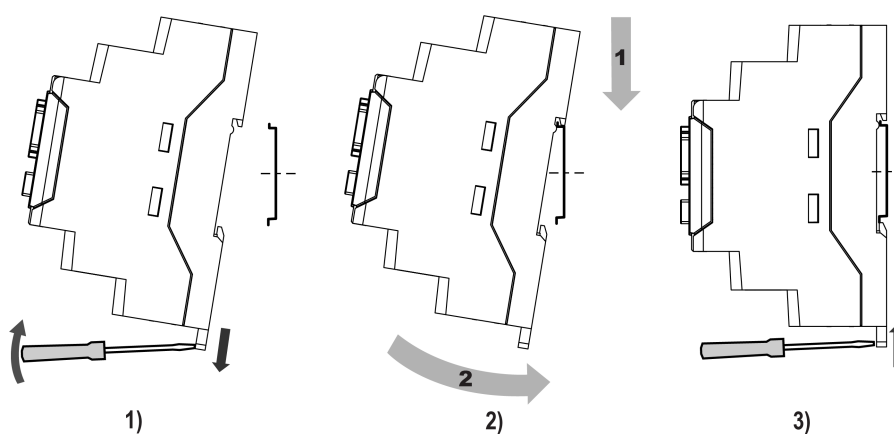
Рисунок 5.2 – Монтаж прибора
