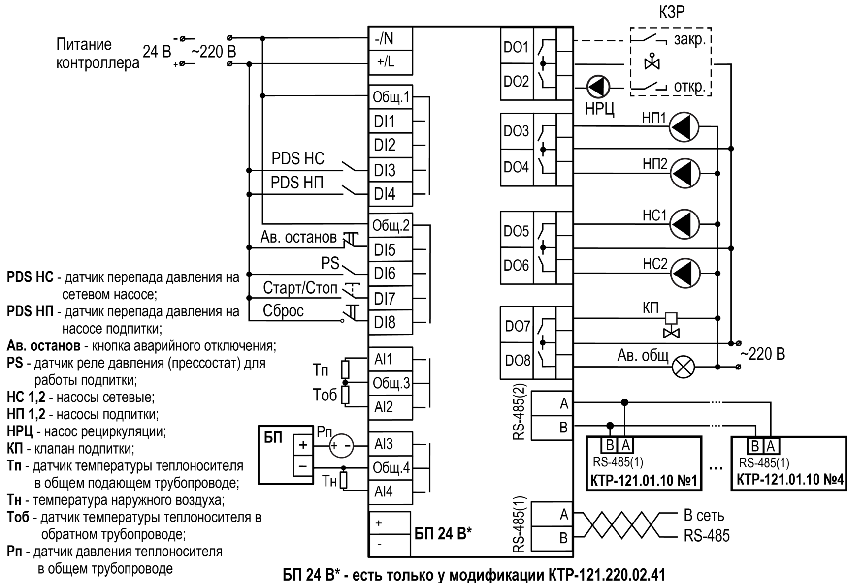
Рисунок 6.4 – Схема подключения
