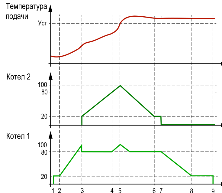
Рисунок 9.6 – Работа модулируемой горелки
