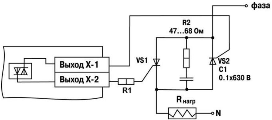
Рисунок Б.11 – Схема подключения нагрузки к ВУ типа С двух тиристор, подключенных встречно-параллельно
