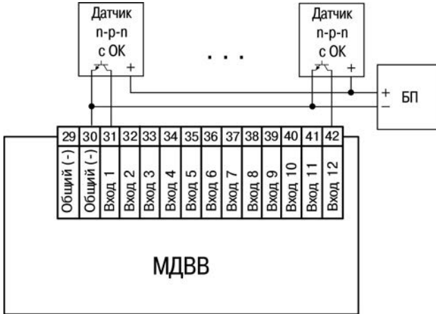
Рисунок Б.7 - Схема подключения дискретных датчиков п-р-п с ОК
