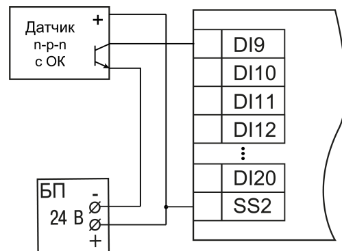
Рисунок 5.11 – Подключение транзисторов типа н-п-п DI9–DI20
