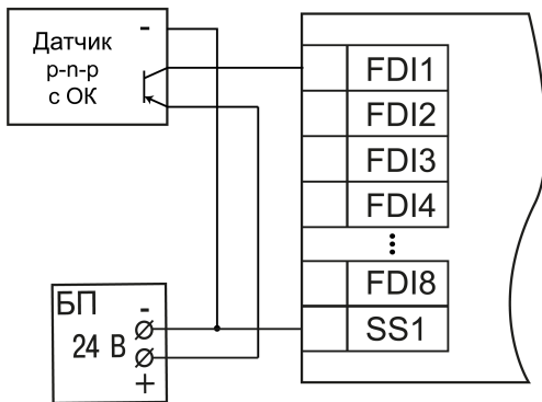
Рисунок 5.8 – Подключение транзисторов типа р-п-п FDI1–FDI8
