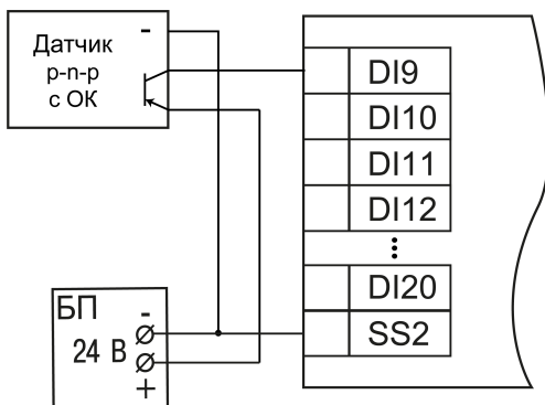
Рисунок 5.10 – Подключение транзисторов типа р-п-п DI9–DI20
