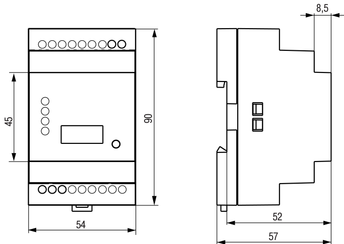
Рисунок 4.2 – Габаритные размеры прибора
