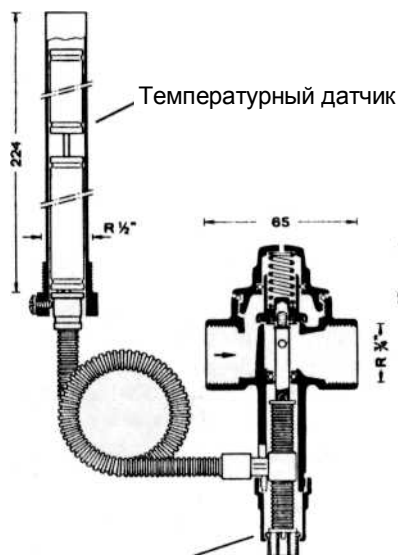
Сильфонная система
