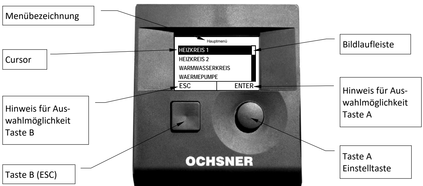
Abbildung 7: Bedienteil MB64xx
