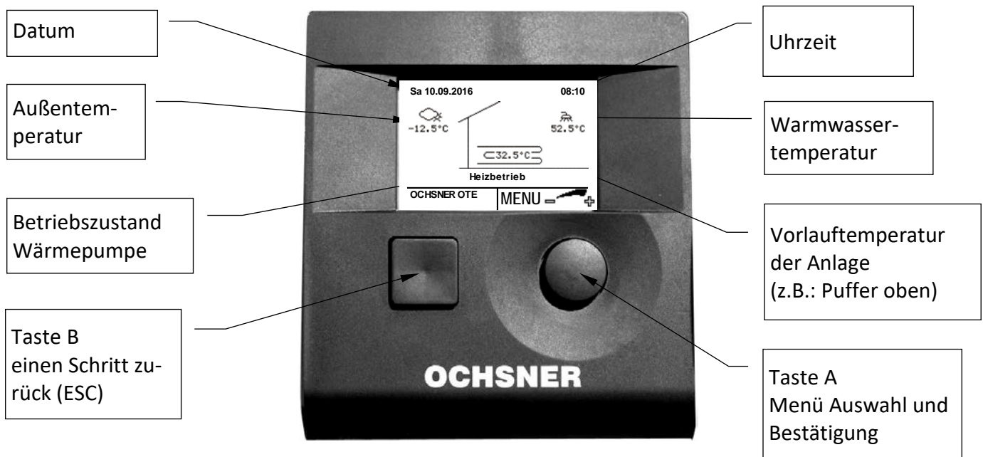
Abbildung 5: Bedienteil MB64xx
