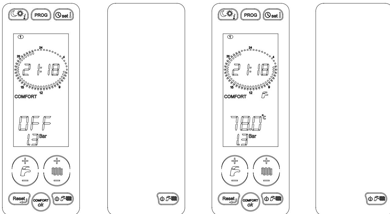
1. РЕЖИМ РАБОТЫ КОТЛА «OFF»
