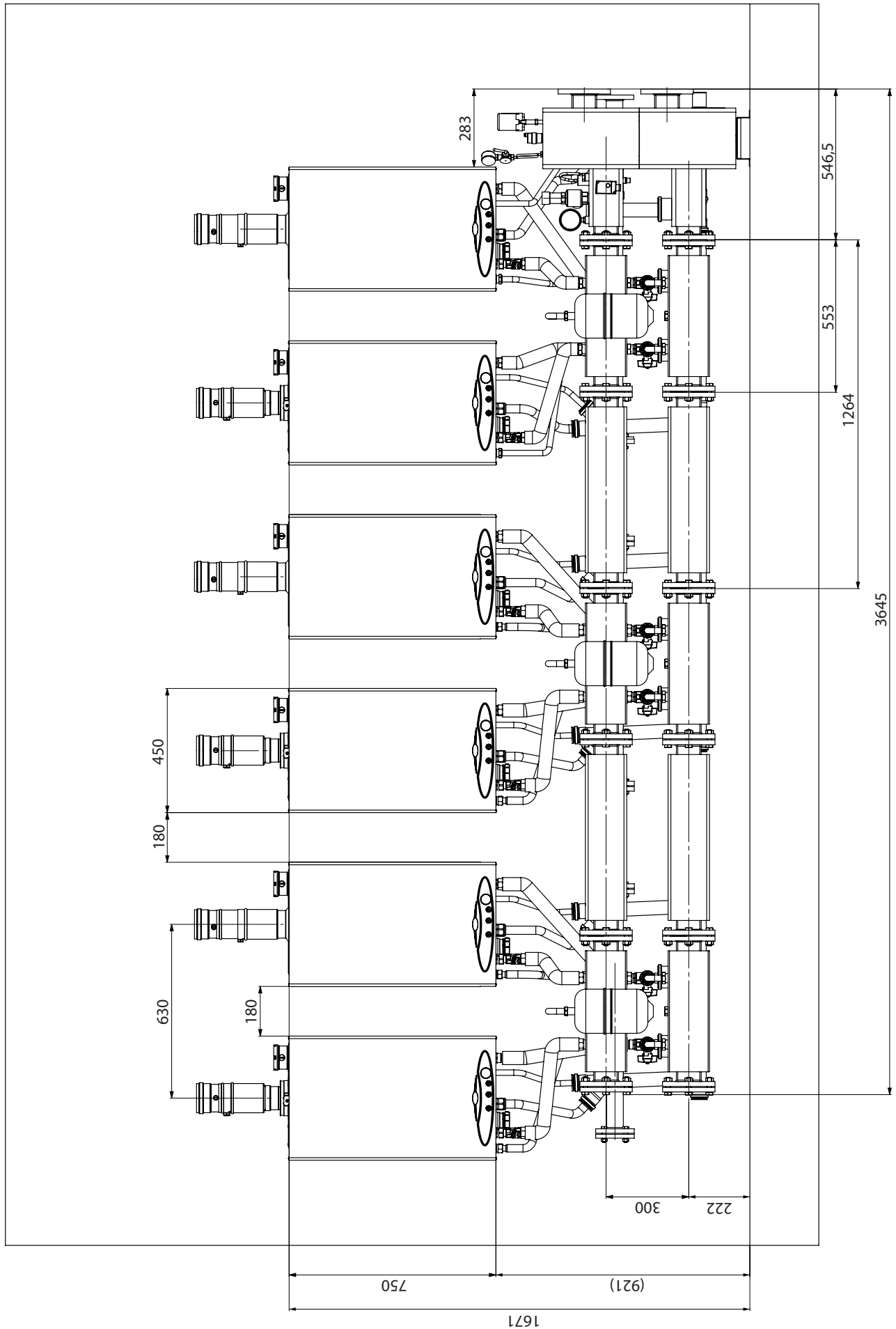
Габариты при правостороннем монтаже модульного теплогенератора на стене. Вид спереди.
