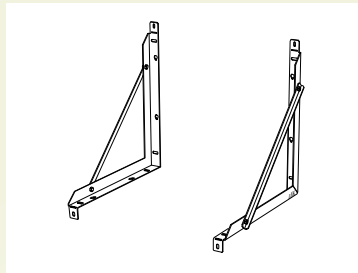
Комплект кронштейнов для модуля FLM Артикул № 067 083
