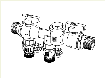
KB R25 Комплект заправочных клапанов Комплект заправочных клапанов для заполнения рассолом шланга коллектора, применяемого в тепловых насосах для горных пород. Включает грязевой фильтр и изоляцию. Артикул № 089 368
