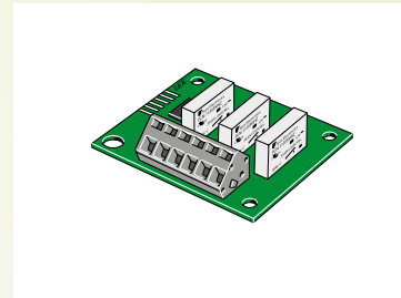
EXC 40 Дополнительная плата релейной цепи При подключении к F1126 геотермального теплового насоса и/или циркуляционного насоса горячей воды требуется дополнительная плата реле. Дополнительная плата реле устанавливается внутри теплового насоса. Артикул № 089 315
