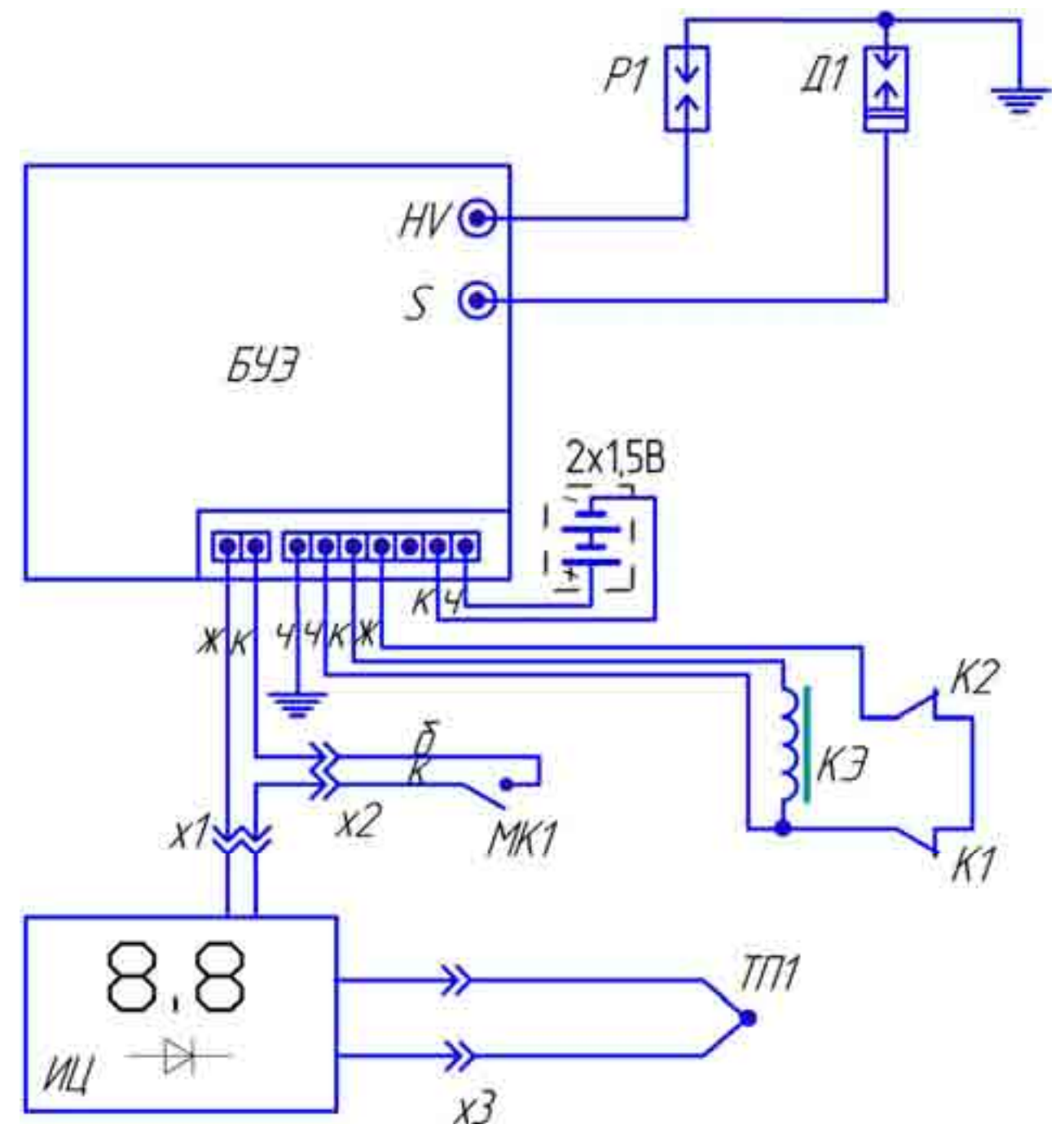
Рисунок 4 Монтажная схема соединений
