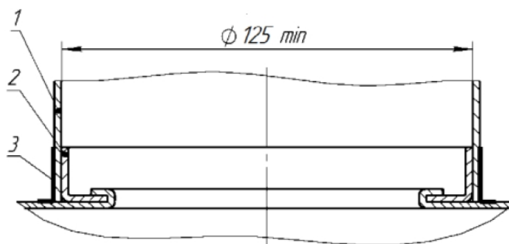
Рисунок 7. Схема подсоединения газоотводящей трубы
