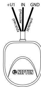
Рис. 6. Маркировка жил.
