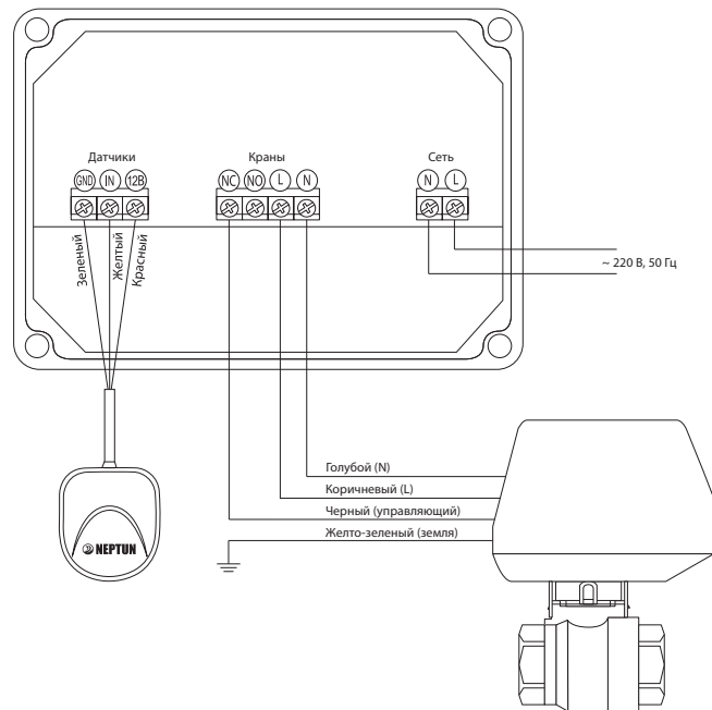
Рис. 9. Схема подключения датчиков и кранов с электроприводом DePala 220 В к модулю управления Neptun Base
