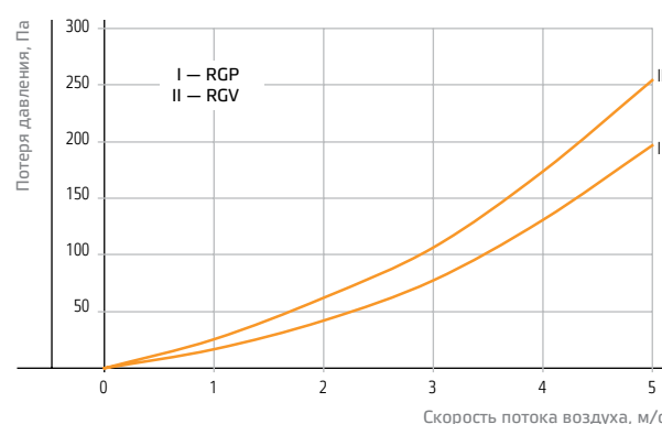
4-рядный гликолевый рекуператор
