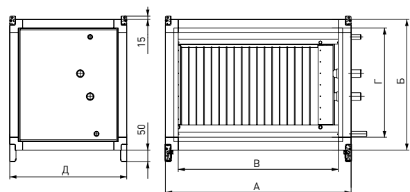
Вытяжная часть рекуператора (RGV)
