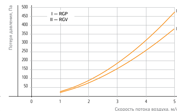
8-рядный гликолевый рекуператор
