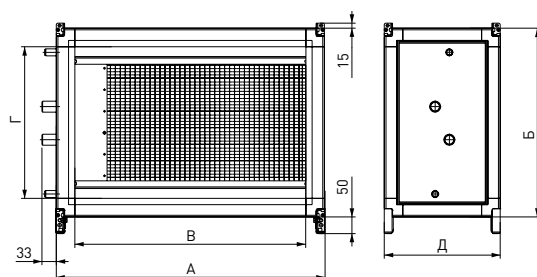
Приточная часть рекуператора (RGP)
