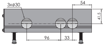
Бок.проекция Размеры подключений Модуль VTМ 145-66
