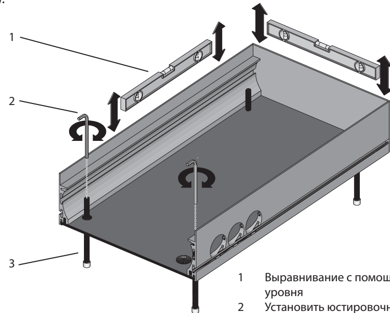
Установить системный конвектор
