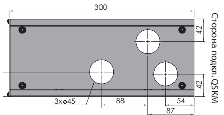
Вид сверху Размеры подключений Модуль VTМN 145-66
