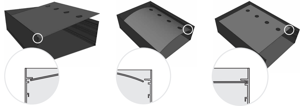
Монтаж непрозрачного покрытия
