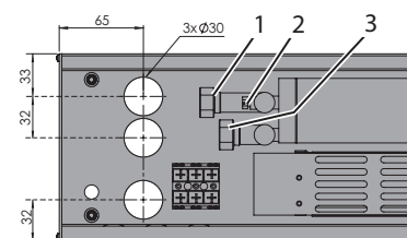
Вид сверху Размеры подключений Сист.конвектор QSKM 145-66
