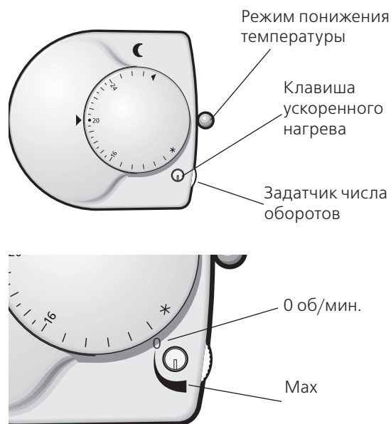
Рис. 1.18. Регулятор «Альфа» с задатчиком скорости (частоты) вращения
