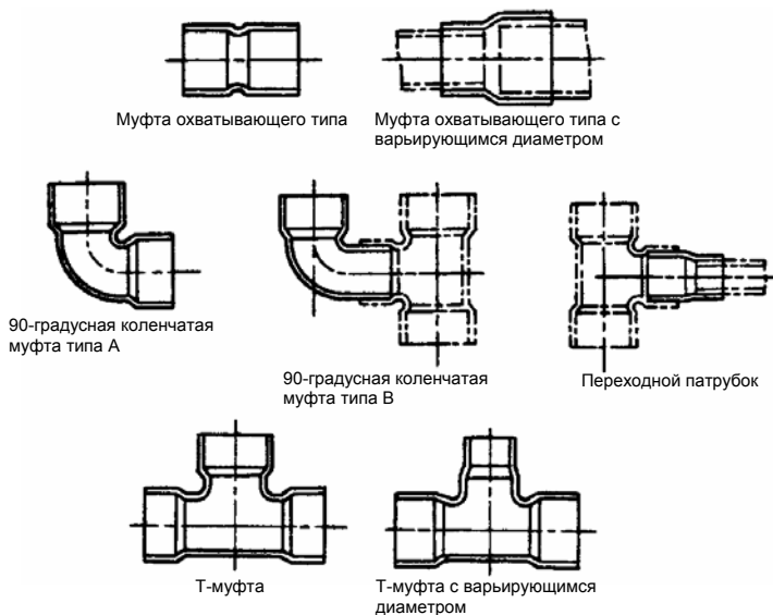
Рис. 2: муфтовые соединения
