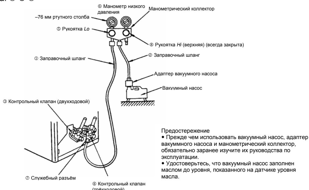
Рис. 6: расположение компонентов во время продувки воздухом с помощью вакуумного насоса
