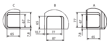
Размеры заглушки
