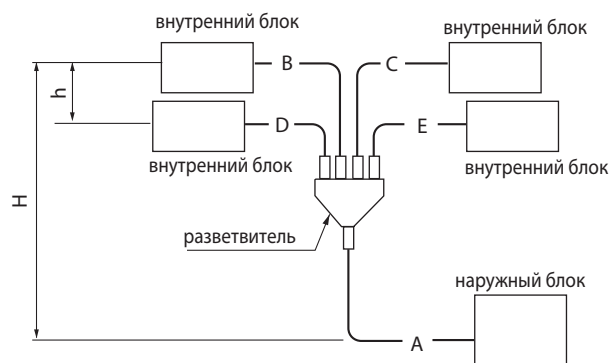
Система 1:4 Суммарная длина: A + B + C + D + E P200, 250 : 70 м
