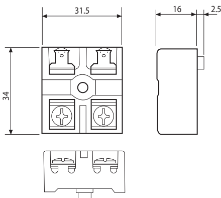
Клеммная колодка
