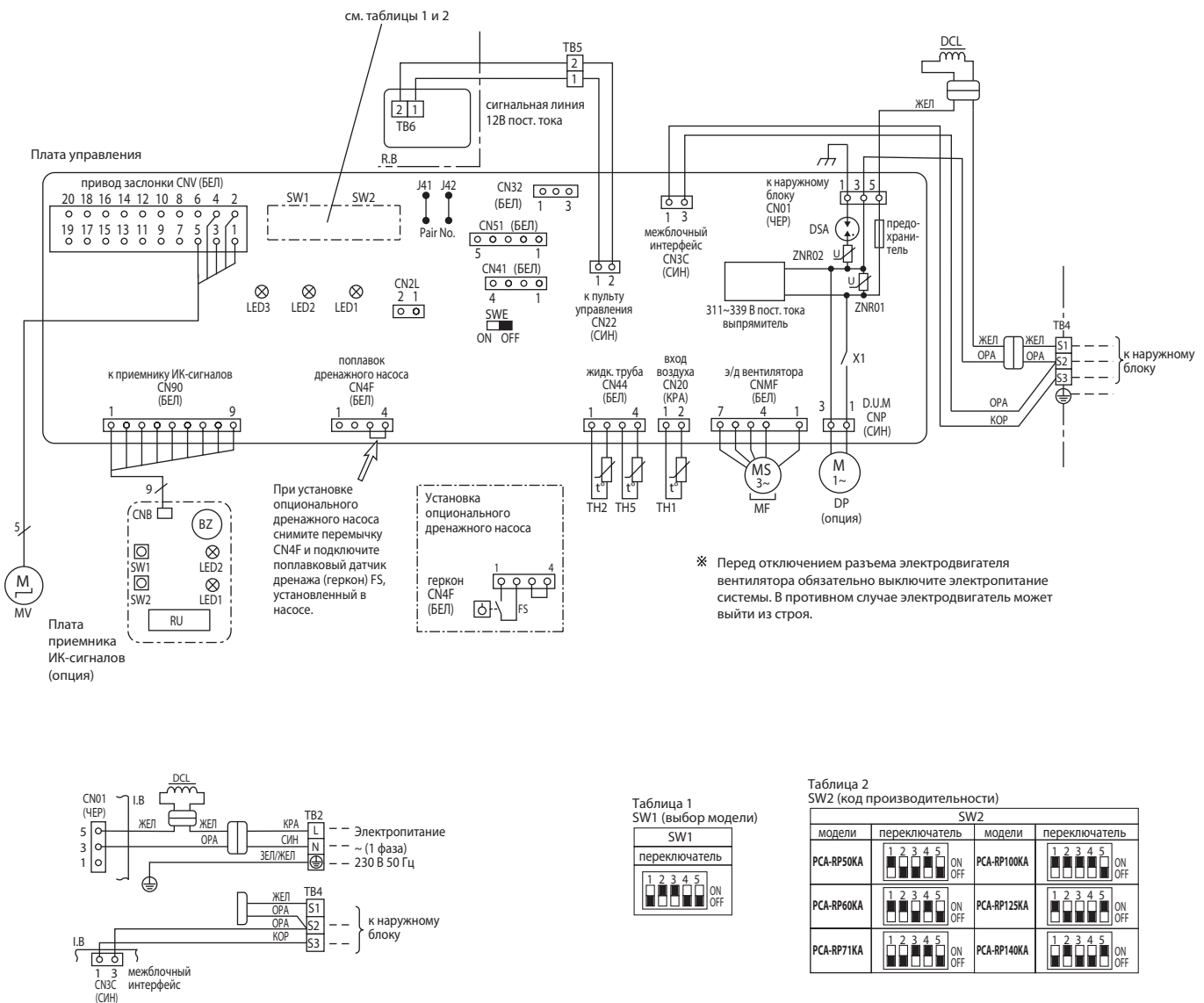
Рис. 1. Раздельное подключение электропитания к наружному и внутренним блокам.
