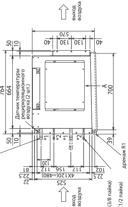
Вид слева
