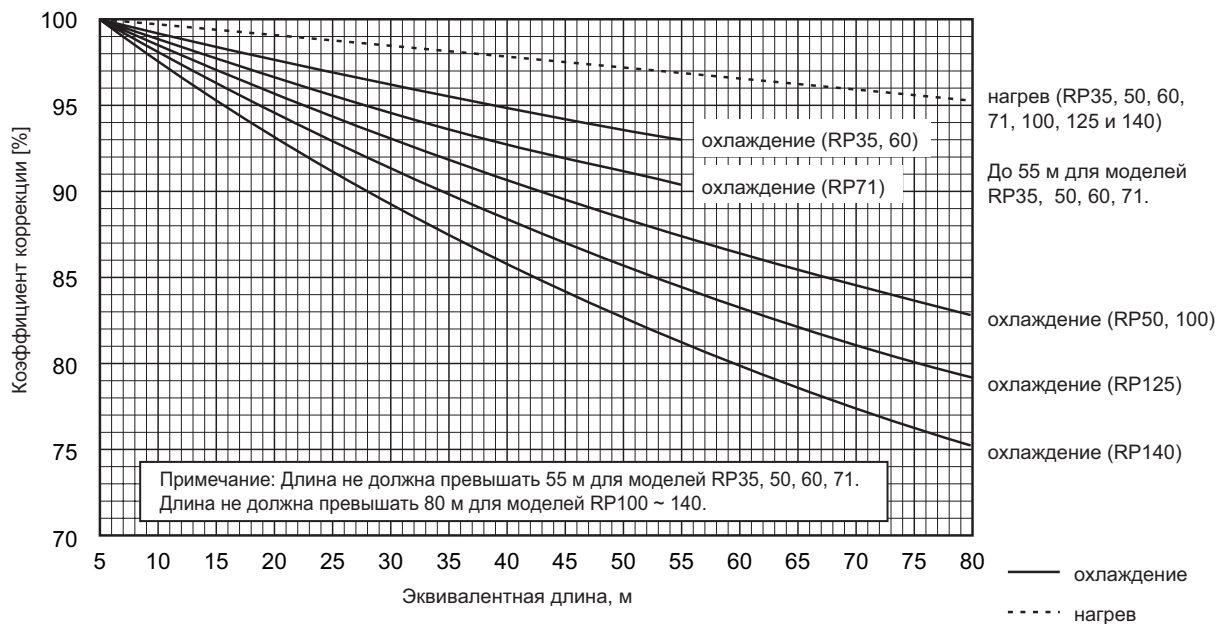
(1) Коррекция производительности PУНЗ-РР · НА2 (стандартный диаметр газовой трубы)
