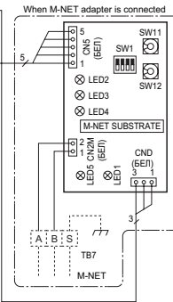
Конвертер для сети M-NET (Сити Мульти)
