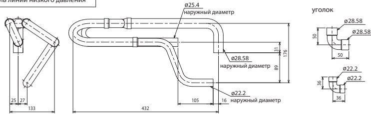
Объединитель труб низкого давления
