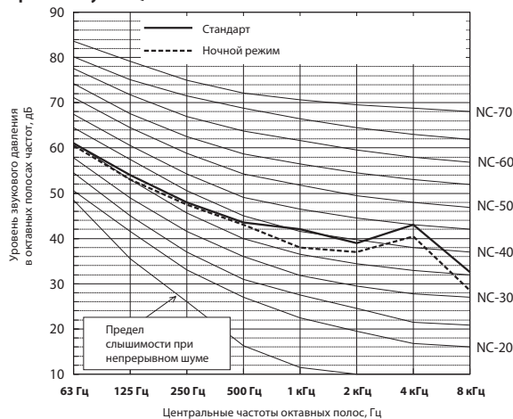
Уровень шума РQНУ-Р250УНМ-А
