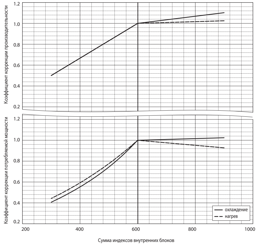
PURY-EP600YSJM-A1
