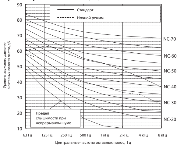
Уровень шума PUHY-P250YJM-A(-BS)
