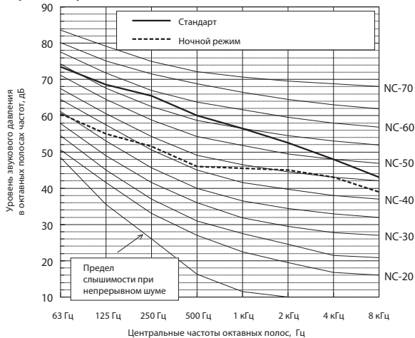
Уровень шума PUHY-EP650YSJM-A(-BS)
