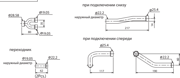
Объединитель линий высокого давления
