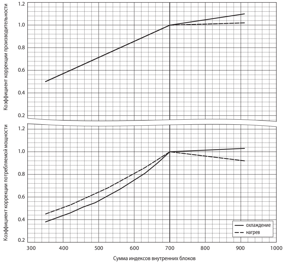
PUHY-P700YSJM-A, PUHY-P700YSJM-A1
