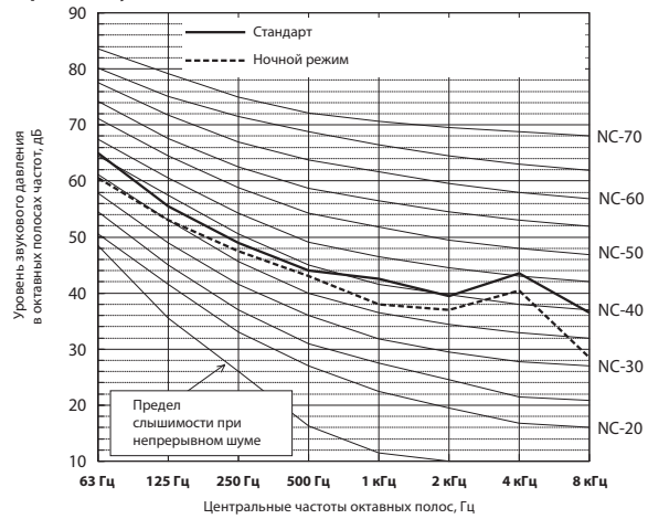
Уровень шума РQНУ-Р300УНМ-А
