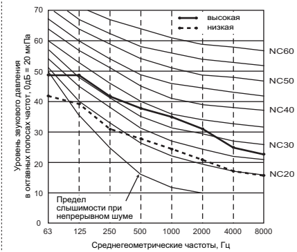
PEFY-P40,50VMH-E Внешнее статическое давление 200Па Электропитание 230,240В, 50/60Гц
