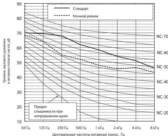
Уровень шума PUHY-P1050YSJM-A(-BS)
