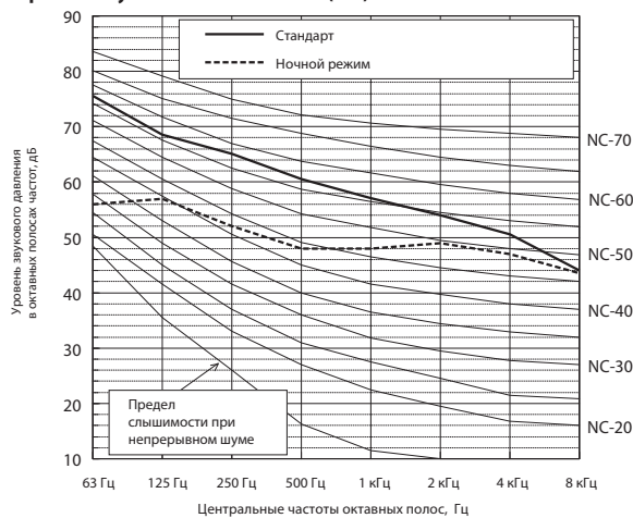
Уровень шума PUHY-P750YSJM-A(-BS)
