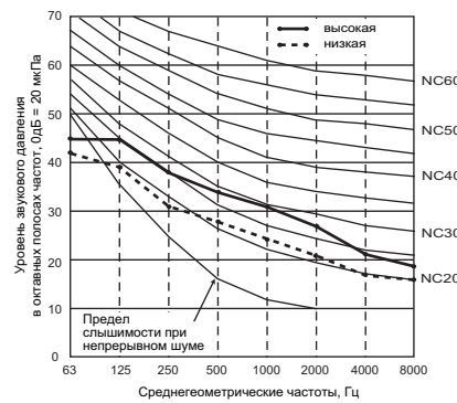
PEFY-P40,50VMH-E Внешнее статическое давление 150Па Электропитание 230,240В, 50/60Гц
