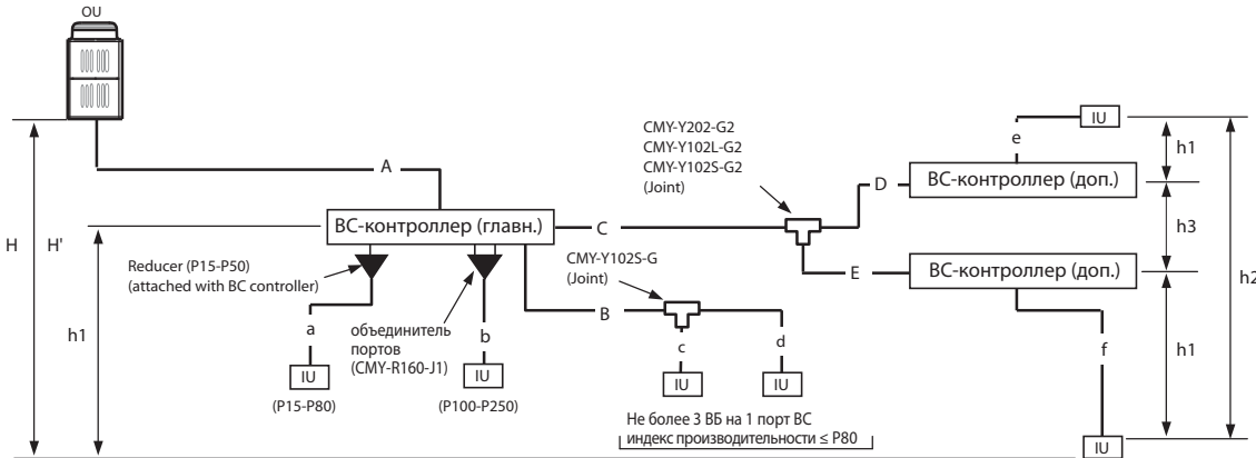
Рис. 6-2-2. Схема фреонопроводов
