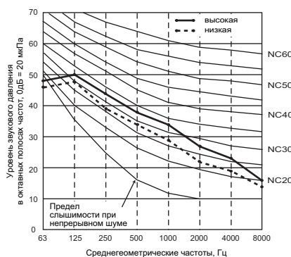
PEFY-P80VMH-E Внешнее статическое давление 100Па Электропитание 220, 230, 240В, 50/60Гц
