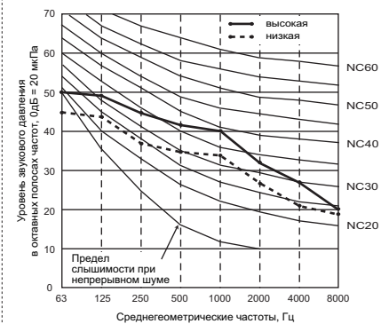
PEFY-P63VMH-E Внешнее статическое давление 200Па Электропитание 230,240В, 50/60Гц
