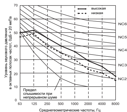
PEFY-P80VMH-E Внешнее статическое давление 150Па Электропитание 230, 240В, 50/60Гц
