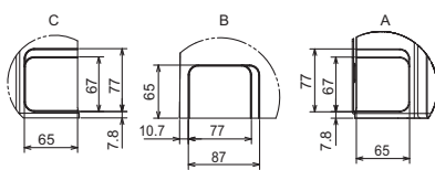
Размеры заглушки
