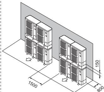
Рис. 13. Установка „один над другим“.
