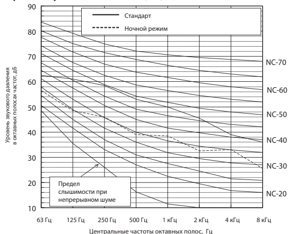
Уровень шума PUHY-P200YJM-A(-BS)
