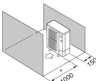
Рис. 4. Препятствие сзади и сбоку.
