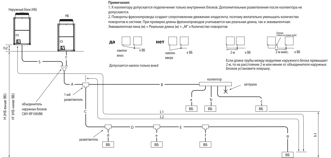
Рис. 4-2. Схема фреонопроводов
