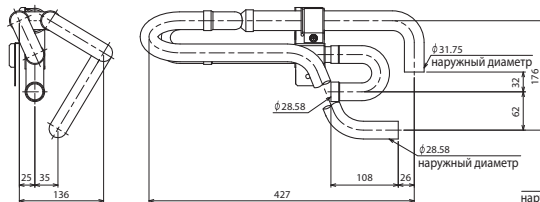
Объединитель линий низкого давления
