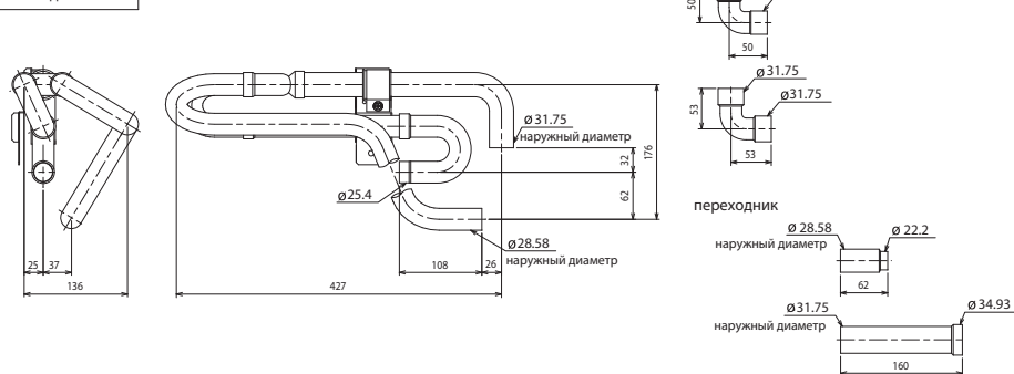
Объединитель линий высокого давления
