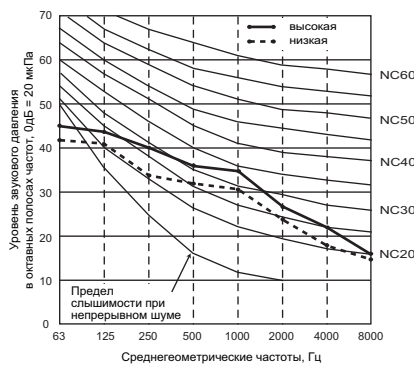
PEFY-P63VMH-E Внешнее статическое давление 100Па Электропитание 230,240В, 50/60Гц
