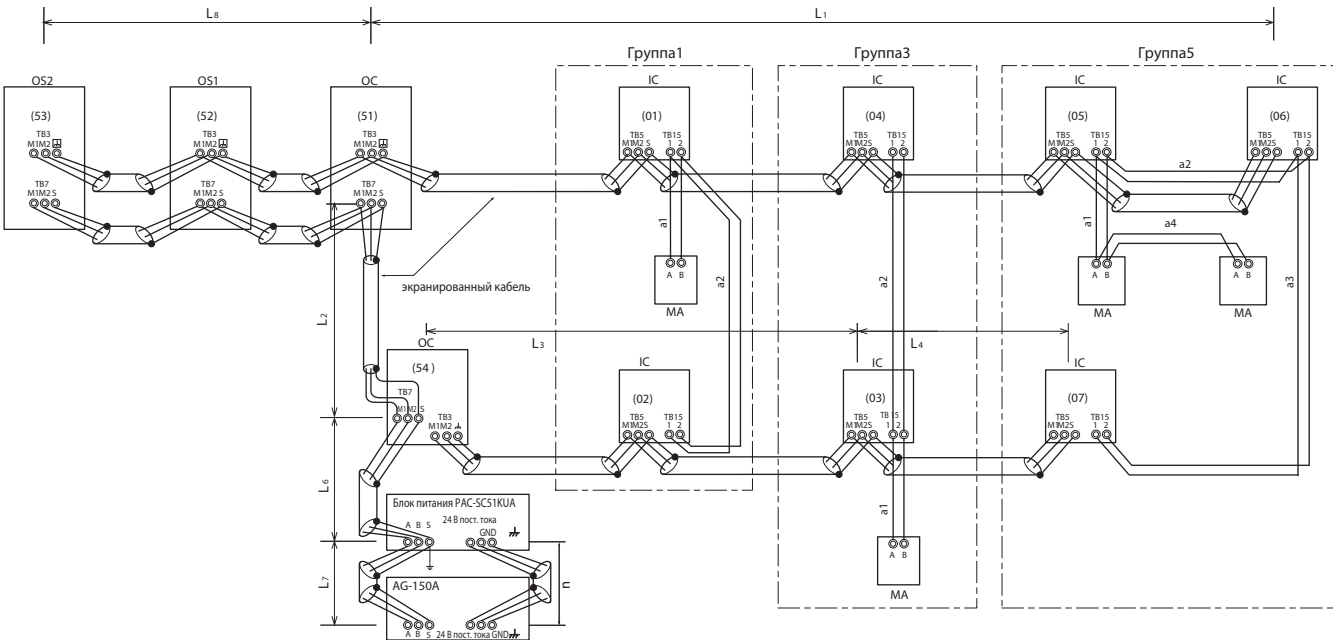
OS, OS1, OS2 : блоки управления наружных приборов; IC: блоки управления внутренних блоков; MA: MA-пульт управления
