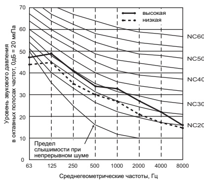
PEFY-P71VMH-E Внешнее статическое давление 100Па Электропитание 230,240В, 50/60Гц
