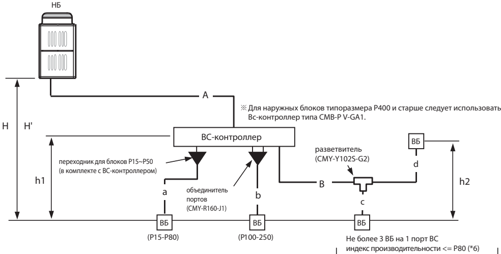
Рис. 5-1A. Схема фреоноводов
