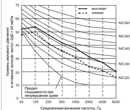
PEFY-P80VMH-E Внешнее статическое давление 200Па Электропитание 230, 240В, 50/60Гц
