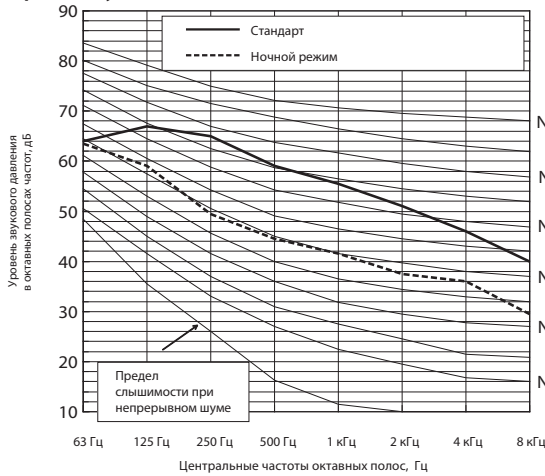
Уровень шума PUHY-RP750YSJM-B(-BS)
