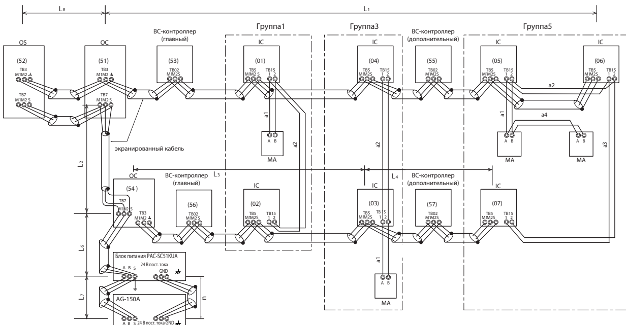
OS, OS: блоки управления наружных приборов; IC: блоки управления внутренних блоков; MA: MA-пульт управления
