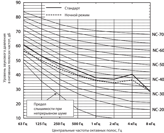
Уровень шума РQНУ-Р200УНМ-А
