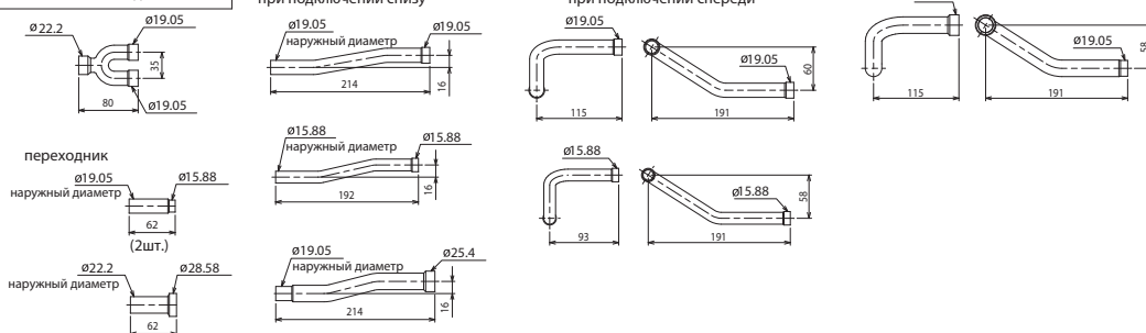
Объединитель линий высокого давления
