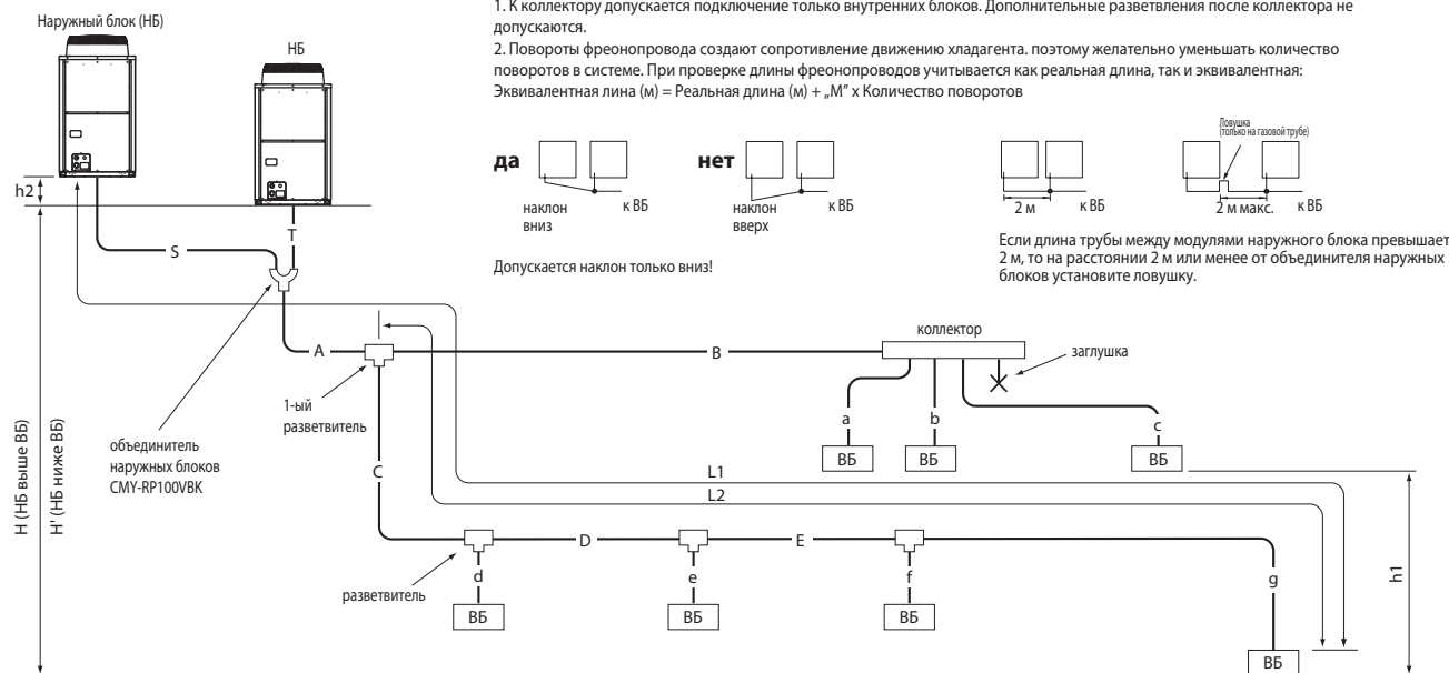
Рис. 4-3. Схема фреонопроводов
