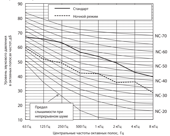
Уровень шума PURY-EP450YSJM-A(-BS)
