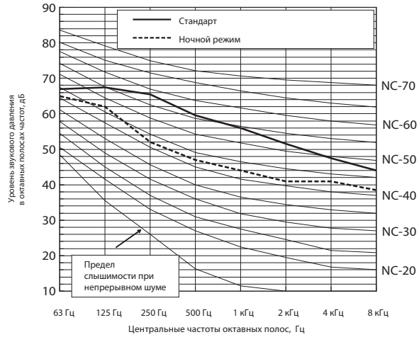
Уровень шума PUHY-RP800YSJM-B(-BS)
