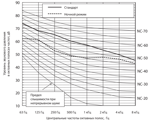
Уровень шума PURY-P700YSJM-A(-BS)
