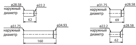
переходник
