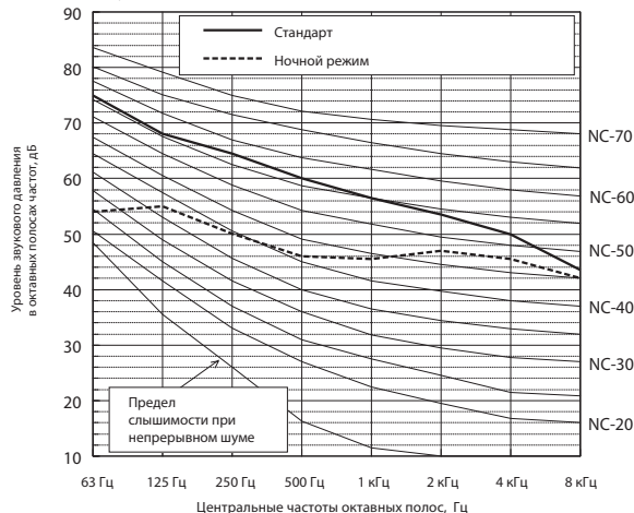
Уровень шума PUHY-P700YSJM-A(-BS)
