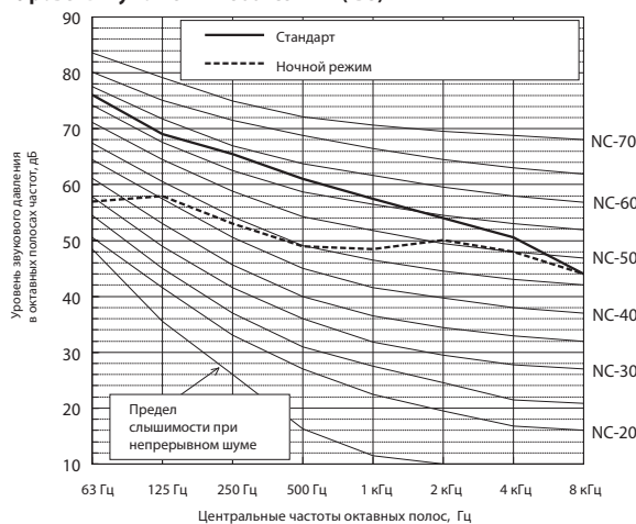
Уровень шума PUHY-P800YSJM-A1(-BS)
