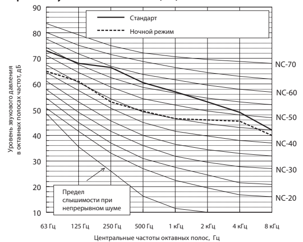
Уровень шума PURY-EP650YSJM-A(-BS)
