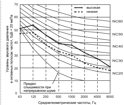
PEFY-P71VMH-E Внешнее статическое давление 200Па Электропитание 230,240В, 50/60Гц
