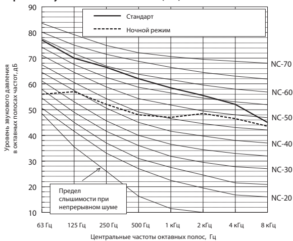
Уровень шума PUHY-EP750YSJM-A1(-BS)
