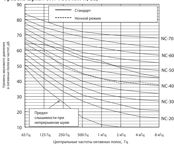
Уровень шума PUHY-P300YJM-A(-BS)
