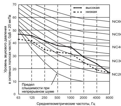
PEFY-P63VMH-E Внешнее статическое давление 150Па Электропитание 230,240В, 50/60Гц
