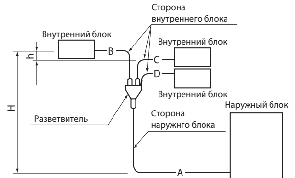
СИСТЕМА С 3 ВНУТРЕННИМИ БЛОКАМИ
