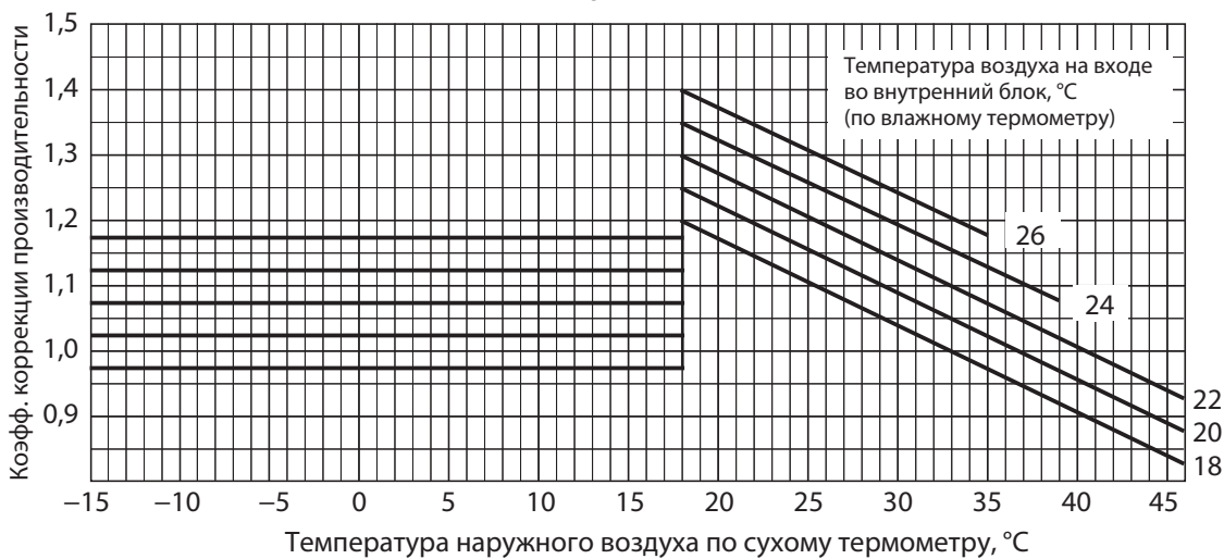
Холодопроизводительность
