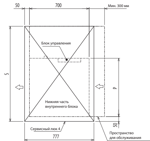
Рис. 5 (Вид по направлению стрелки В)
