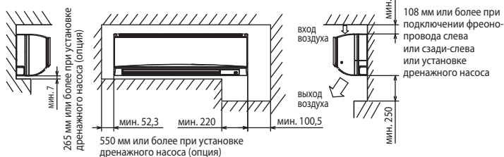
Необходимое пространство для установки внутреннего блока
