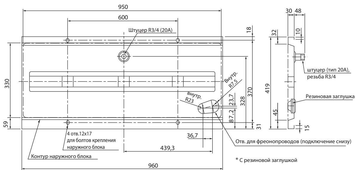
Фронтальная часть блока
