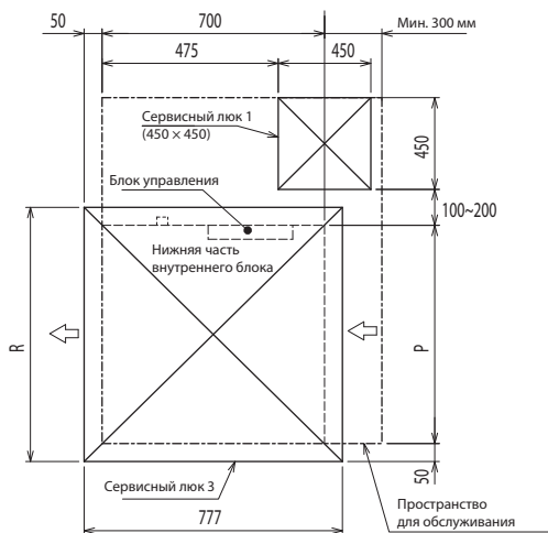
Рис. 4 (Вид по направлению стрелки В)
