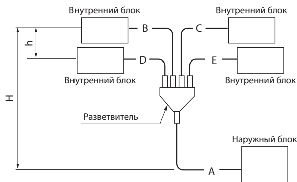
СИСТЕМА С 4 ВНУТРЕННИМИ БЛОКАМИ
