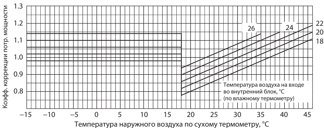
Потребляемая мощность (режим охлаждения)
