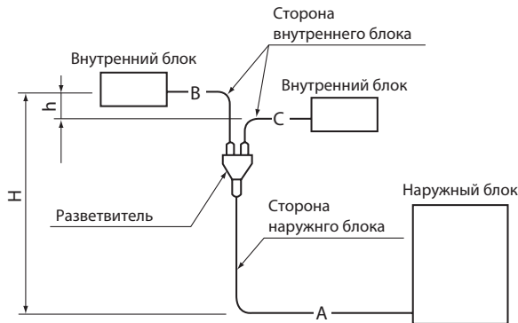
СИСТЕМА С 2 ВНУТРЕННИМИ БЛОКАМИ
