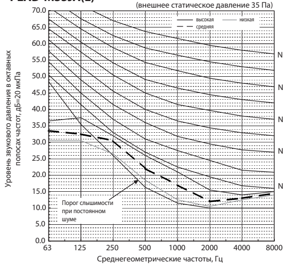
PEAD-M35JA(L)
