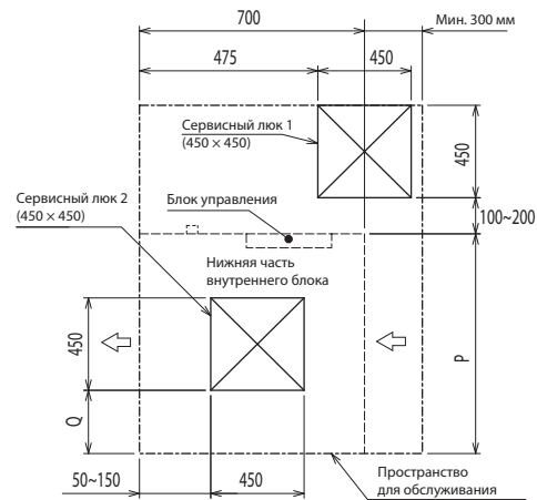
Рис. 2 (Вид по направлению стрелки А)
