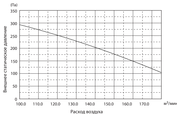
PEA-RP500GAQ
