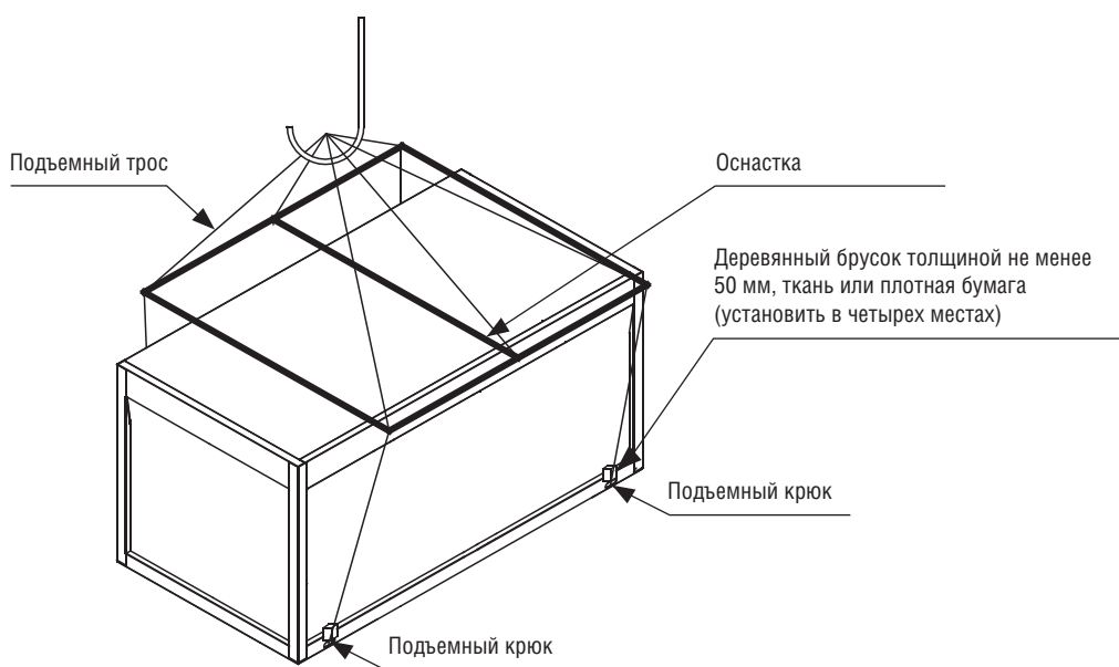
Рис. 2-1. Подъем модуля
