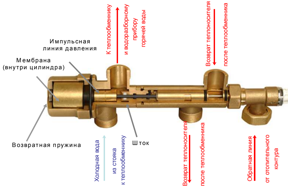
Рис. 3. Трехходовой РМ-регулятор.
