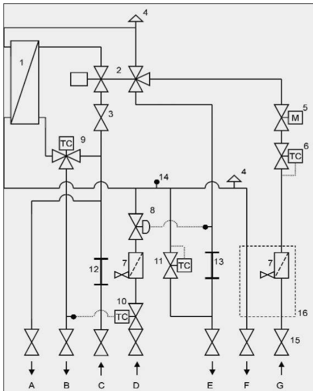
Рис. 1 Гидравлическая схема станции Logotherm
