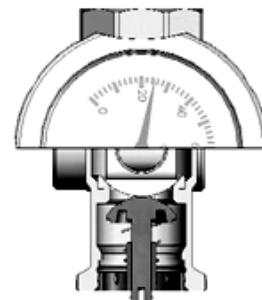
Шаровый кран закрыт
