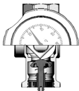
Обратный клапан «открыт», шаровый кран открыт
