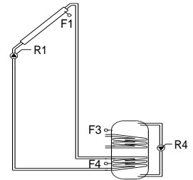
Дополнительная схема с Гидравлической схемой 1
