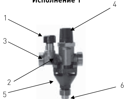
Исполнение 1"
