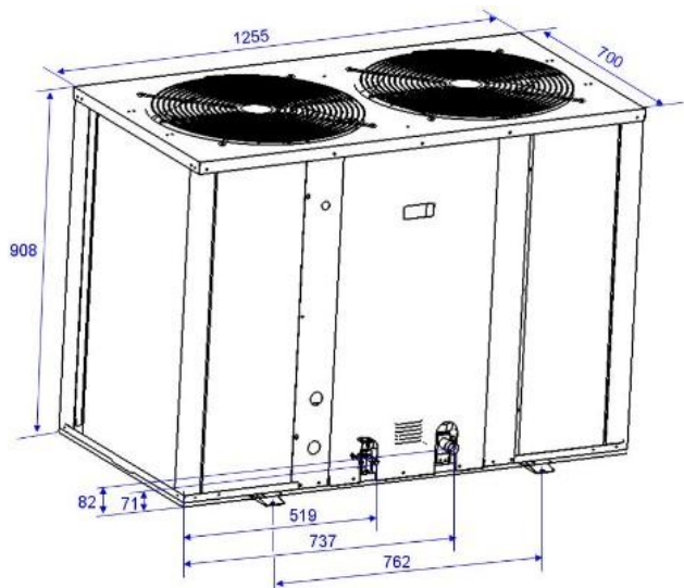
35kW
