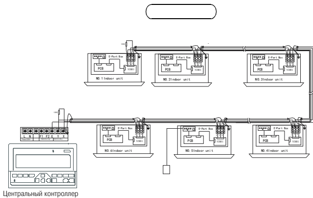
Центральный контроллер
