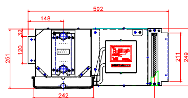
Воздухозаборная камера с фильтром (забор воздуха сзади)
