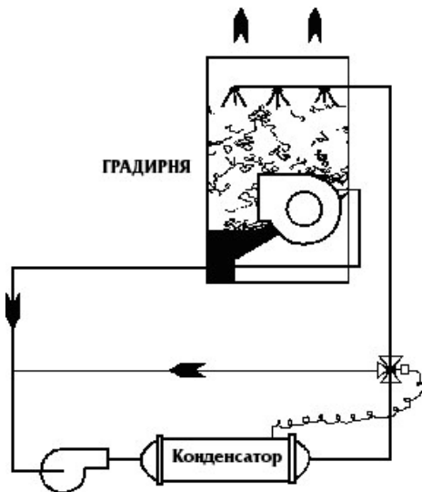
Рис. 2. Клапан байпасирования градирни
