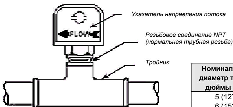
Рис. 4 – Реле протока
