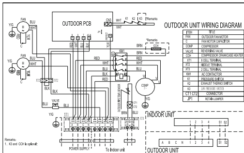
Схема для наружных блоков (Модель LAC-60T-OUT)
