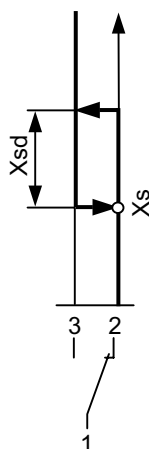
Изображение 2: Установка точек переключения датчика сигналов давления
