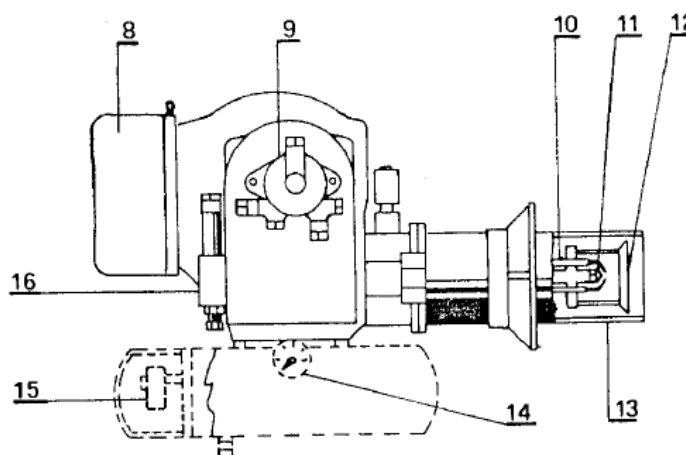
Рис. 2 Горелки типа PG и PN
