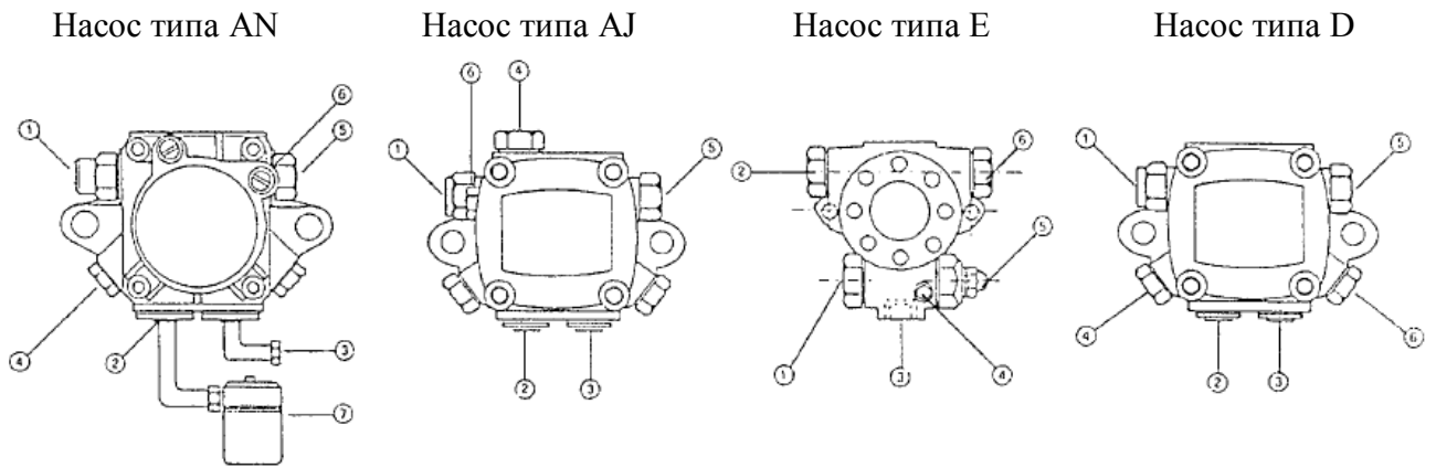
Рис. 6 Гидравлические соединения
