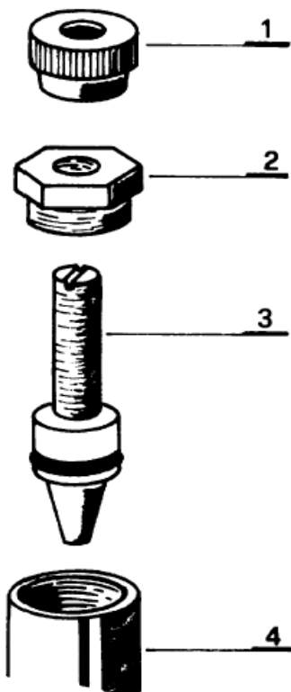
Рис. 22 Демпфирующий клапан
