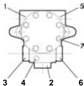
Насос типа SUNTEC E7
