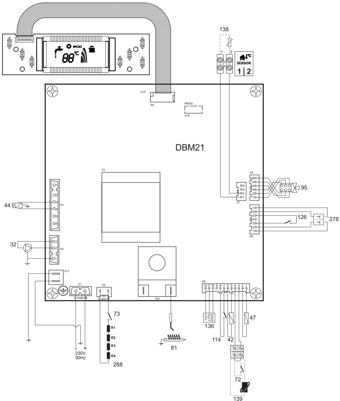
рис. 25 - Электрическая схема
