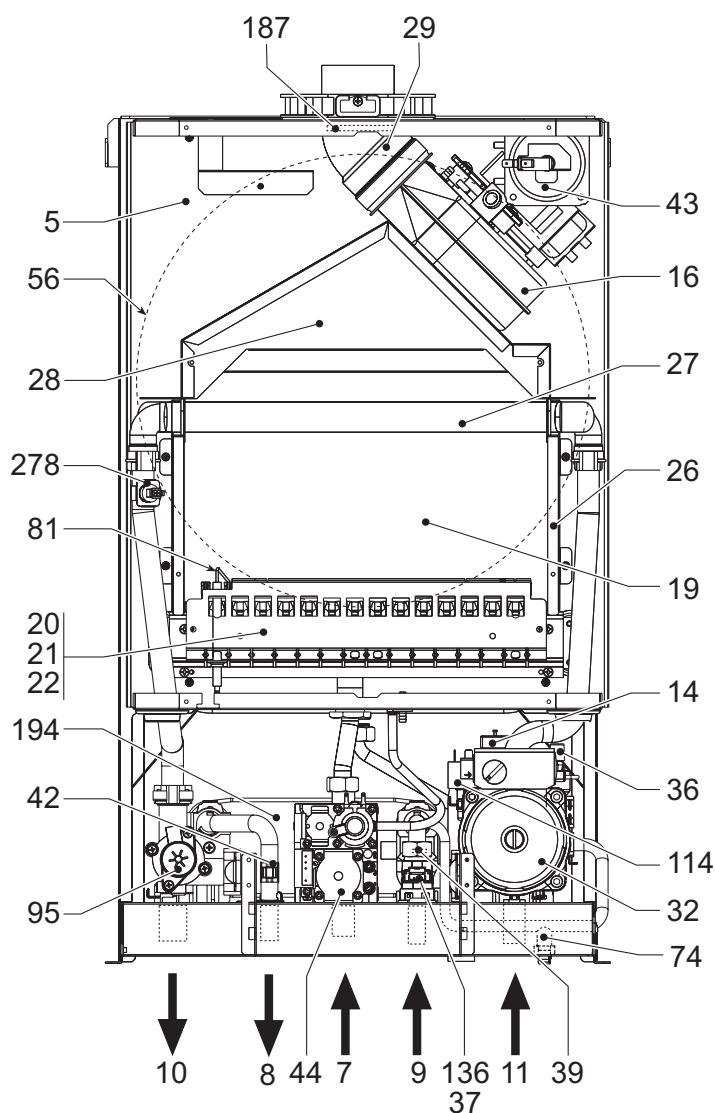
рис. 27 - Общий вид
