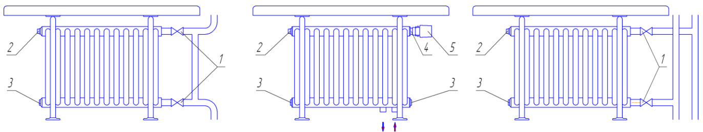
Однотрубная система
