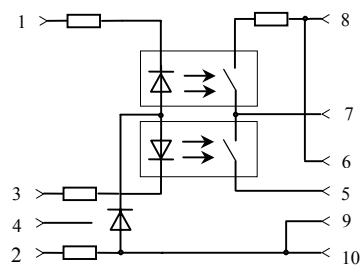
Рисунок 4 – Схема модуля МС-02
