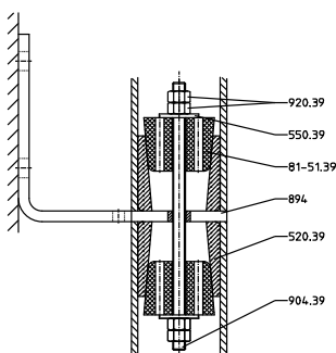
Рисунок 13: Монтаж центрального крепления
