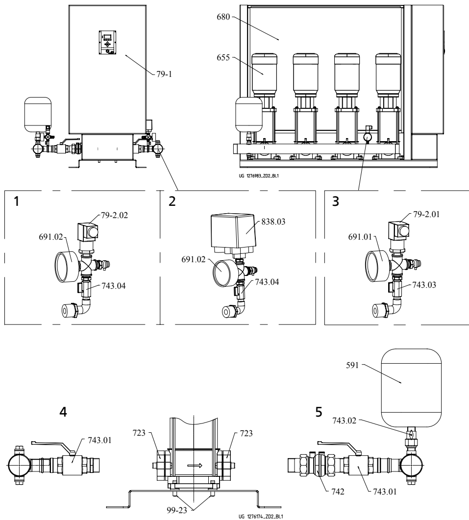
Рисунок 13: Запасные части для Hyamat V с Movitec 2, 4, 6, 10, 18
