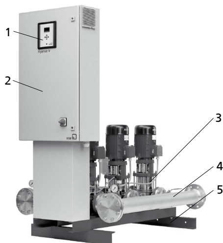
Рисунок 3: Внешний вид Hyamat V
