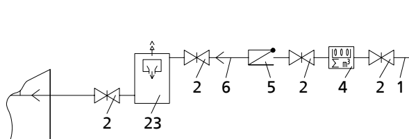
Рисунок 16: Технологическая схема, опосредованное подключение
