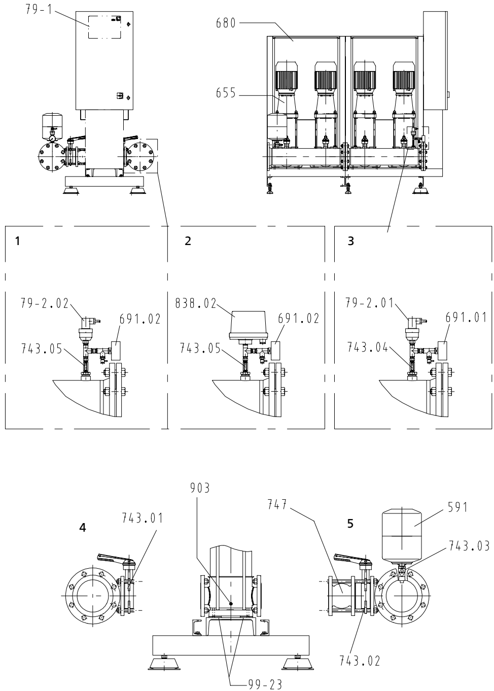
Рисунок 14: Запасные части для Hyamat V с Movitec 32, 45, 65, 90
