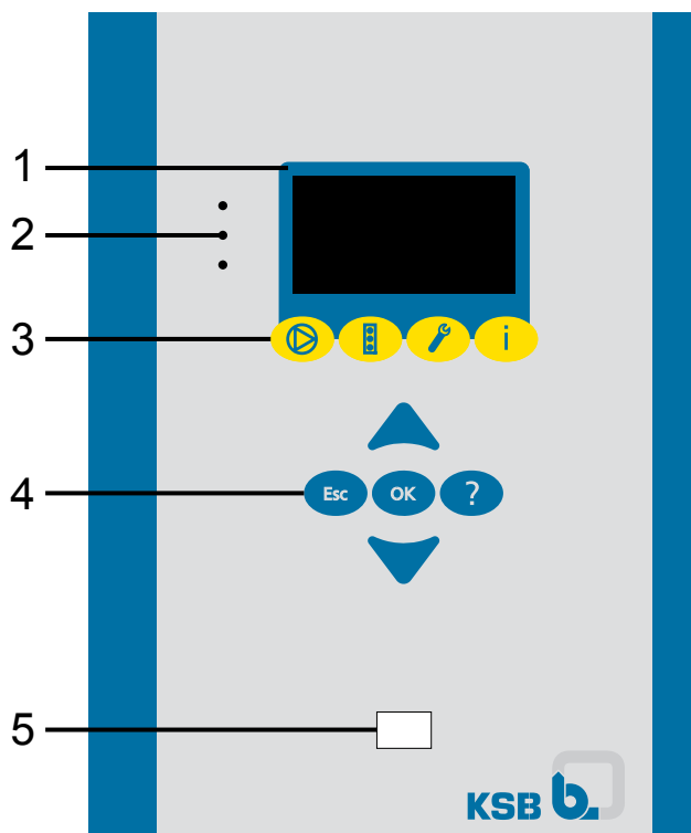
Рисунок 6: Панель управления BoosterControl Advanced
