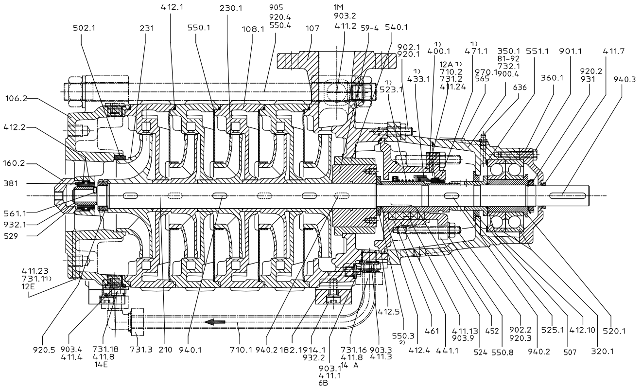
Рисунок 51: Multitec - тип компоновки А - типоразмер 65-100
