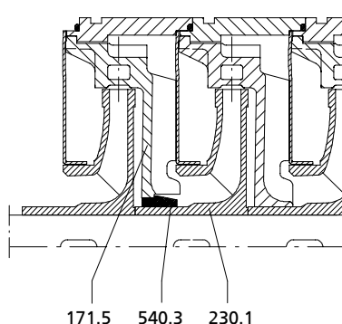
Рисунок 40: Втулка (промежуточная опора)
