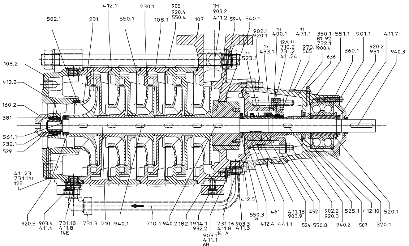
Рисунок 50: Multitec - тип компоновки А - типоразмер 32-50
