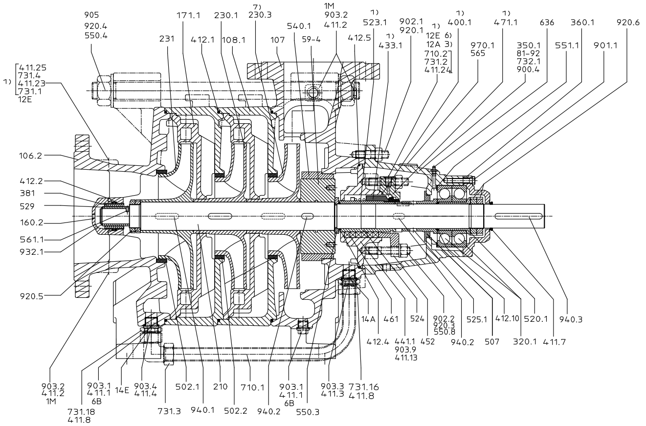
Рисунок 52: Multitec - тип компоновки А - типоразмер 125-150
