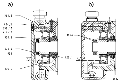
Рисунок 27: Масляная смазка и лабиринтное уплотнение: а) Multitec 32-125 и б) Multitec 150
