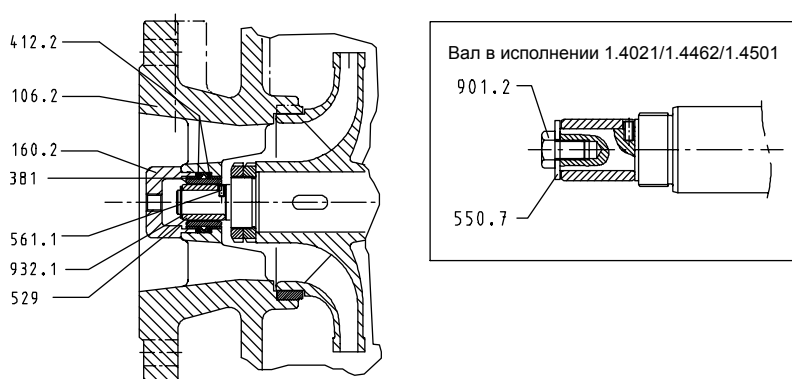
Рисунок 21: Демонтаж подшипников скольжения - аксиальный всасывающий патрубков
