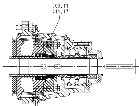
Рисунок 19: Резьбовая пробка отверстия для удаления воздуха уплотнительной камеры (уплотнительная камера с водяным охлаждением) - типоразмер с 125 по 150 (и при необходимости для типоразмеров 32-100 как специальное оборудование)
