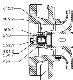
Рисунок 22: Демонтаж подшипника скольжения - аксиальный всасывающий патрубков (Multitec-RO)
